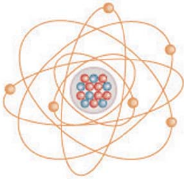
Carbono 14 inestable (radiactivo)
