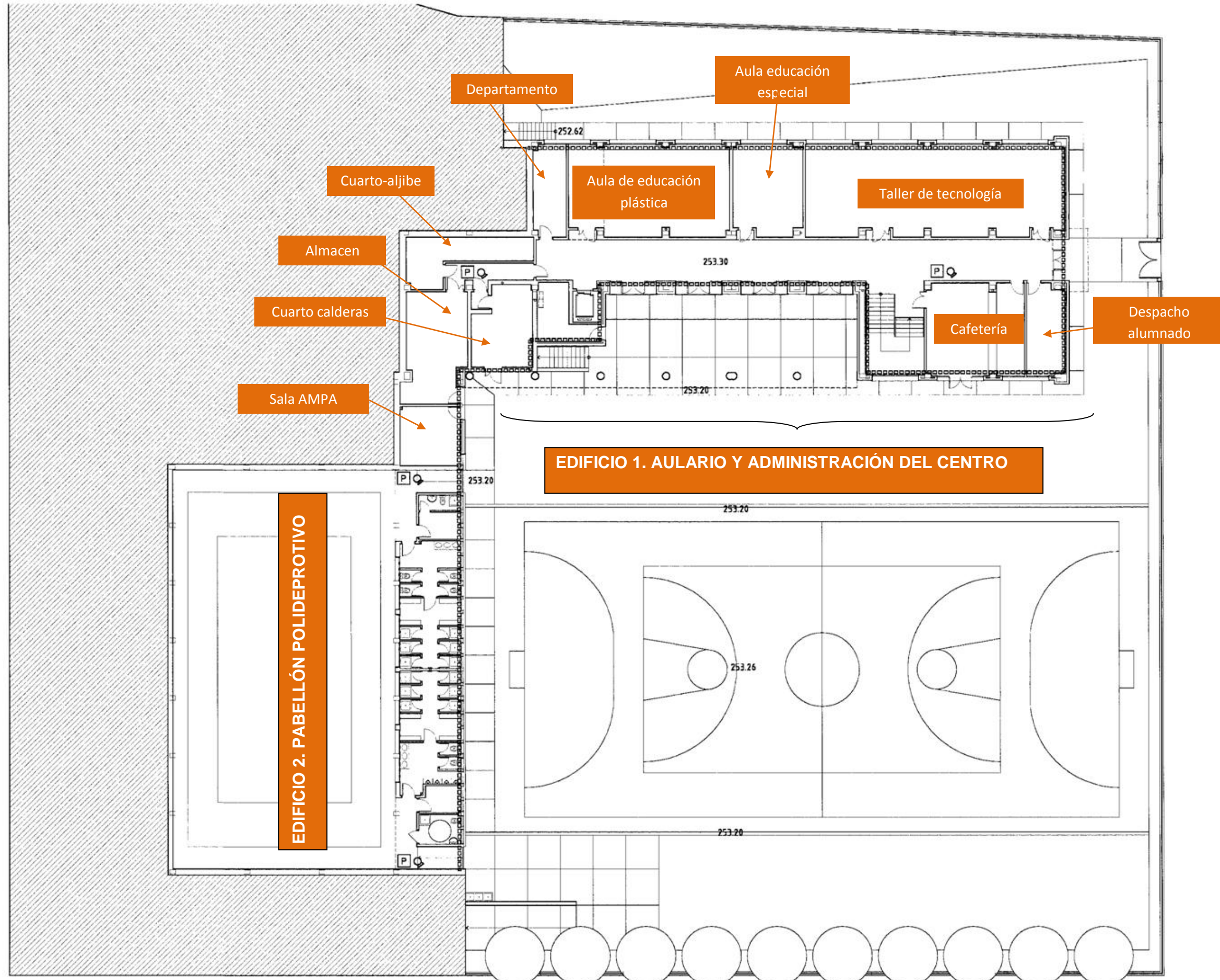
PLANO Nº 3A (Plano descriptivo de planta. Planta 0)
