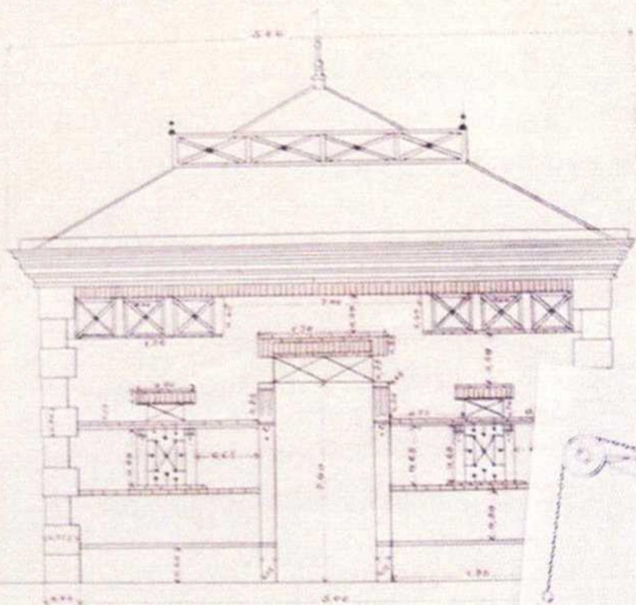
Fachada principal. Escala de 1:50.
