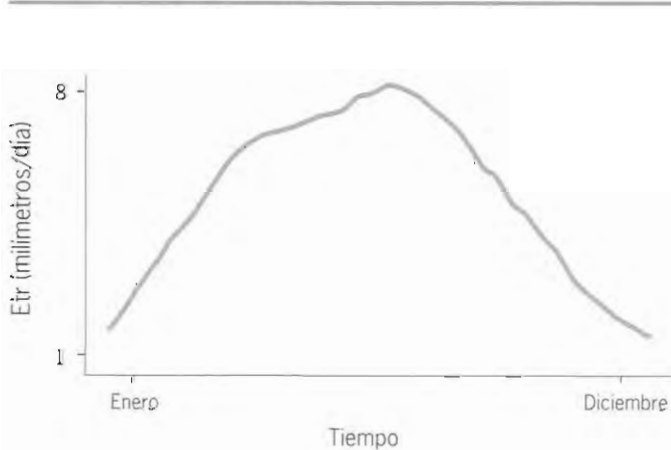
Figura 3. Curva típica de evapotranspiración de referencia (ETr)
