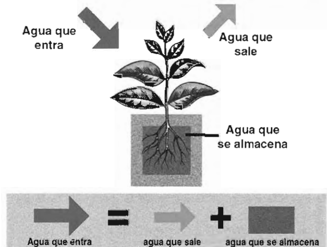
Figura 8. Balance de agua en el sistema suelo-planta
