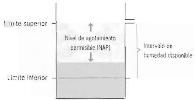
Figura 6. Representación esquemática del Nivel de Agotamiento Permissible
