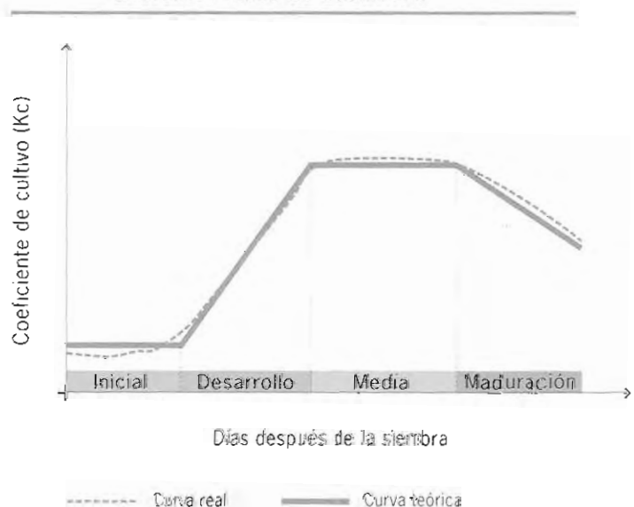
Figura 4. Curvas real y teórica típicas de coeficiente de cultivo para especies anuales, según las diferentes fases de desarrollo
