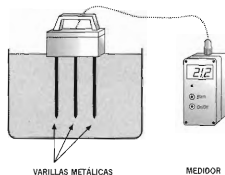
Figura 8. Esquema de un TDR
