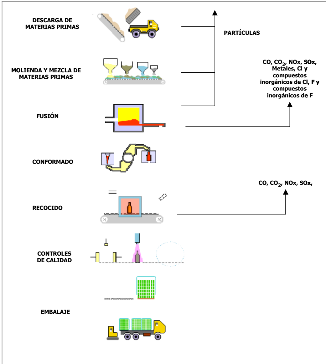
Figura 1. Diagrama del proceso de fabricación y emisiones asociadas
