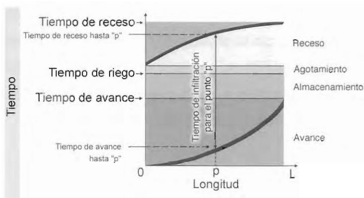
Figura 10. Fases del riego por superficie, tiempos característicos y representación del tiempo de infiltración
