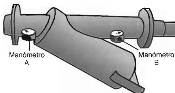
Figura 2. Determinación de la diferencia de presión existente a la entrada y a la salida de un filtro de malla.
