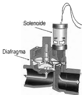
Figura 4. Representación esquemática de una electroválvula
