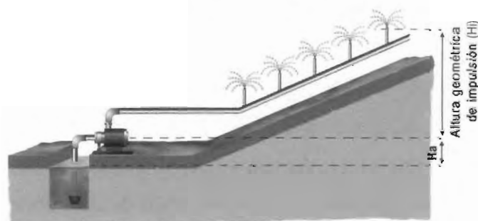
Figura 7. Representación esquemática de la altura geométrica de impulsión.
