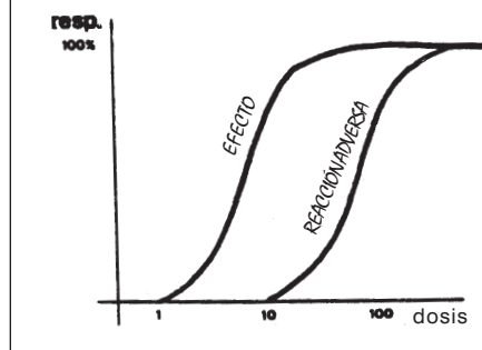
Fig. 10: Curva dosis-respuesta
