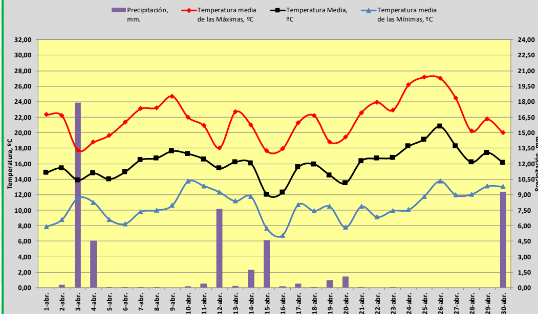
TEMPERATURA Y PRECIPITACIÓN. ABRIL DE 2025. MÁLAGA
