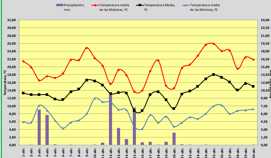
TEMPERATURA Y PRECIPITACIÓN. ABRIL DE 2025. GRANADA
