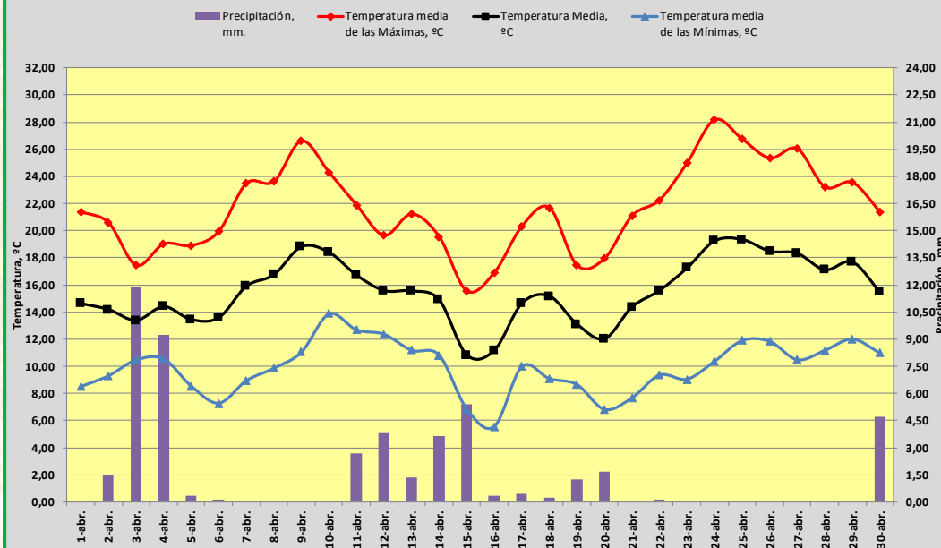
TEMPERATURA Y PRECIPITACIÓN. ABRIL DE 2025. ANDALUCÍA
