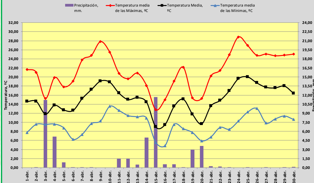
TEMPERATURA Y PRECIPITACIÓN. ABRIL DE 2025. JAÉN
