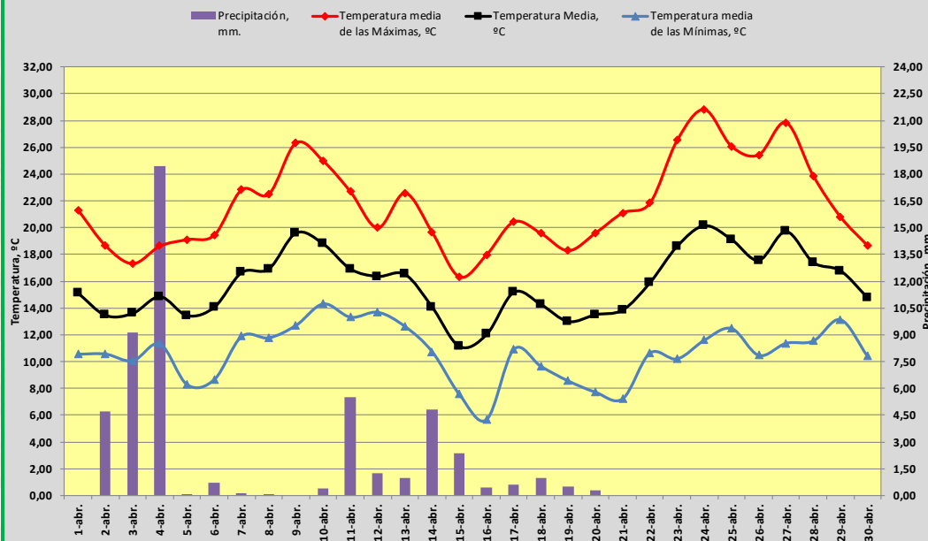
TEMPERATURA Y PRECIPITACIÓN. ABRIL DE 2025. HUELVA
