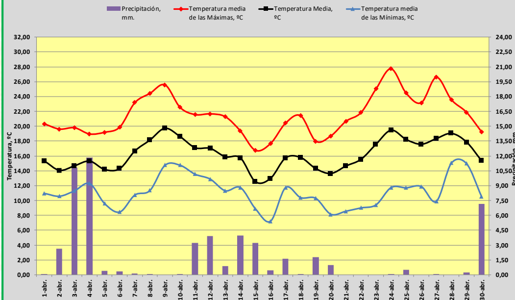
TEMPERATURA Y PRECIPITACIÓN. ABRIL DE 2025. CÁDIZ
