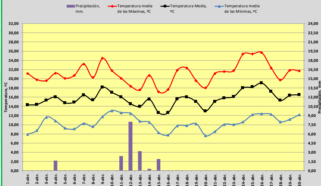
TEMPERATURA Y PRECIPITACIÓN. ABRIL DE 2025. ALMERÍA
