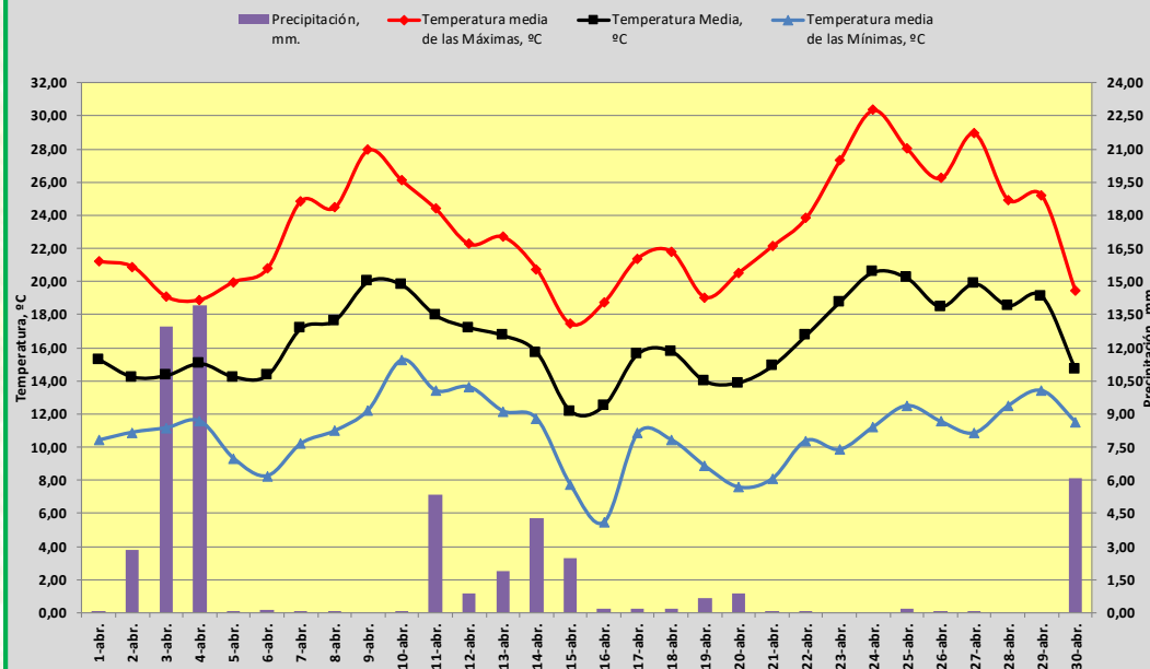
TEMPERATURA Y PRECIPITACIÓN. ABRIL DE 2025. SEVILLA
