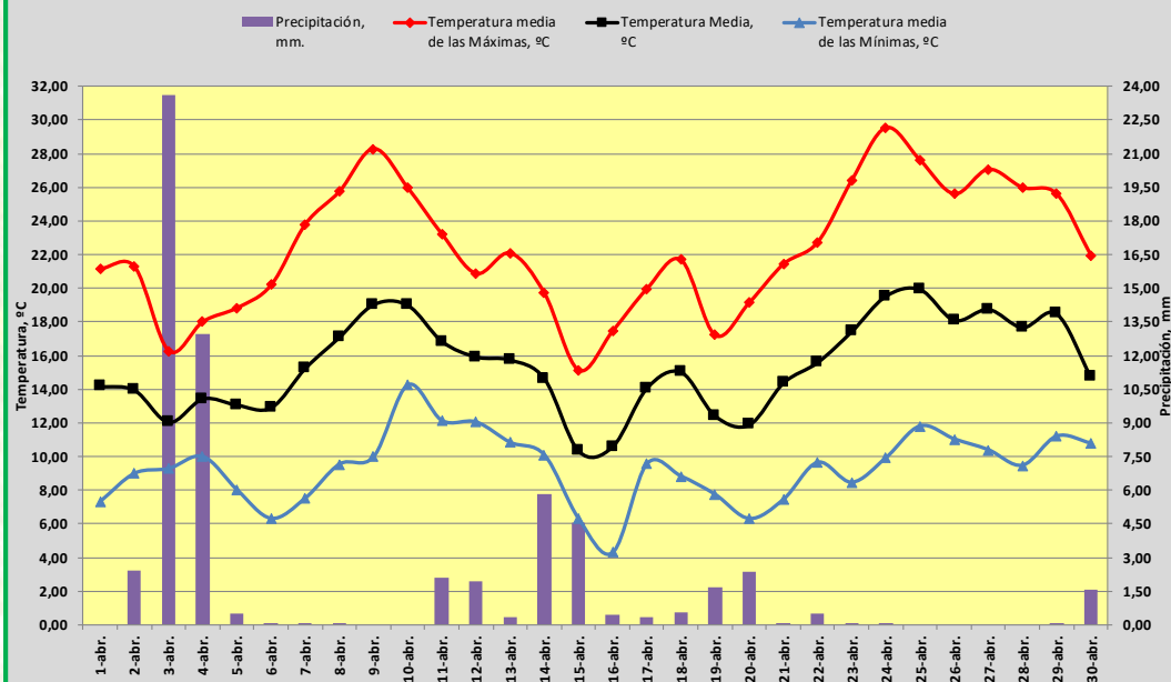
TEMPERATURA Y PRECIPITACIÓN. ABRIL DE 2025. CÓRDOBA
