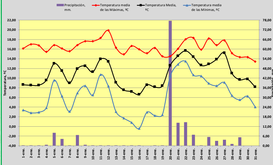
TEMPERATURA Y PRECIPITACIÓN. ENERO DE 2025. HUELVA
