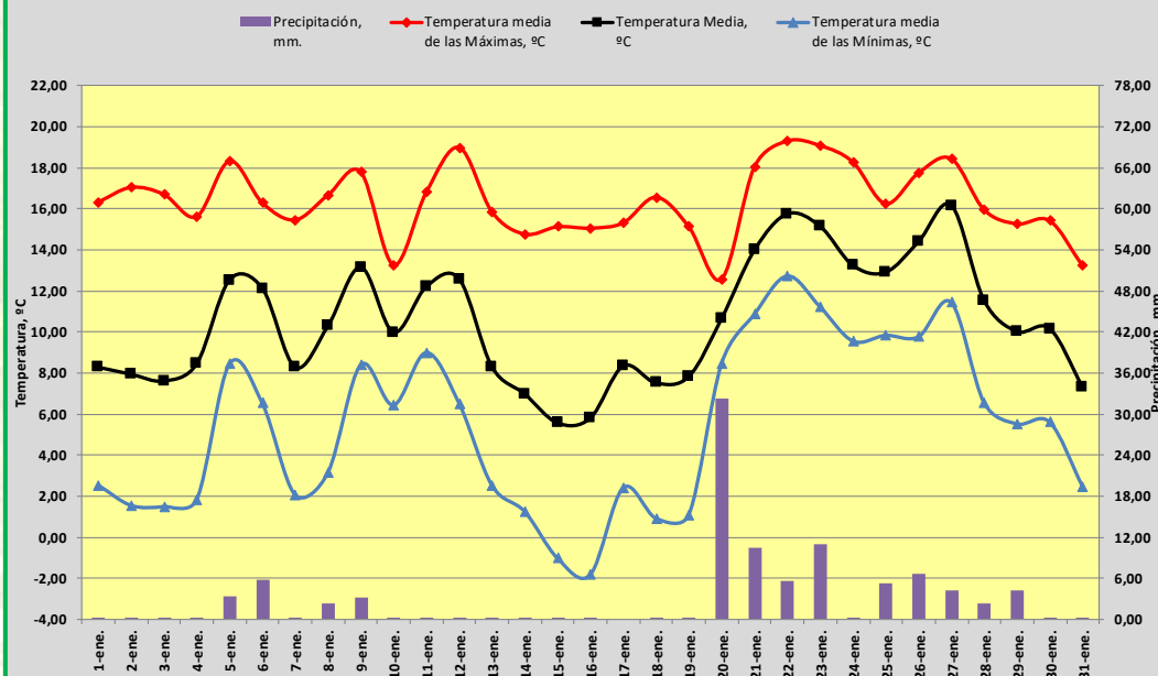
TEMPERATURA Y PRECIPITACIÓN. ENERO DE 2025. SEVILLA
