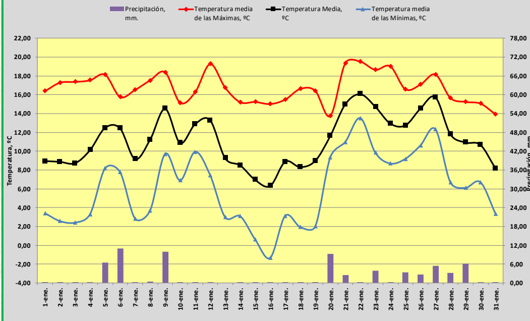
TEMPERATURA Y PRECIPITACIÓN. ENERO DE 2025. CÁDIZ
