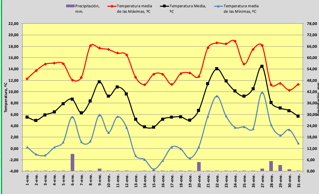
TEMPERATURA Y PRECIPITACIÓN. ENERO DE 2025. GRANADA
