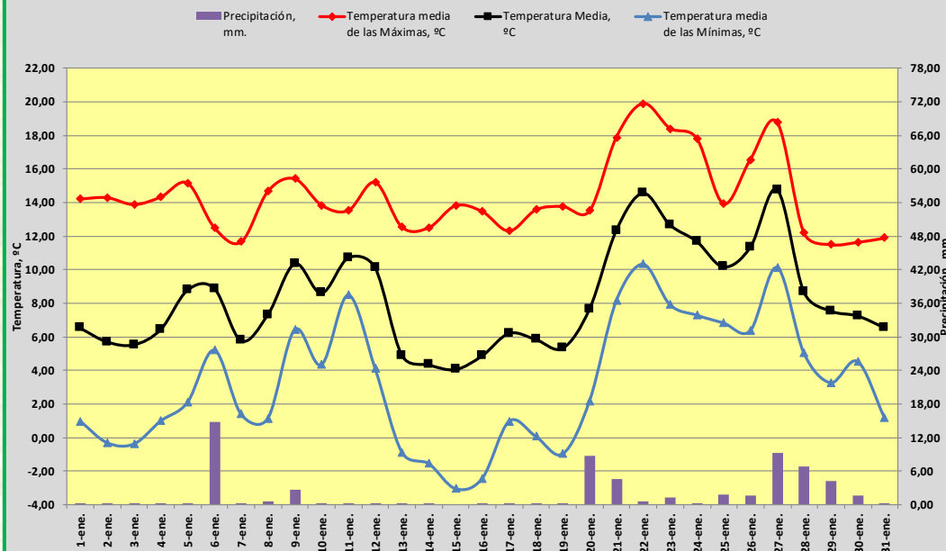
TEMPERATURA Y PRECIPITACIÓN. ENERO DE 2025. JAÉN
