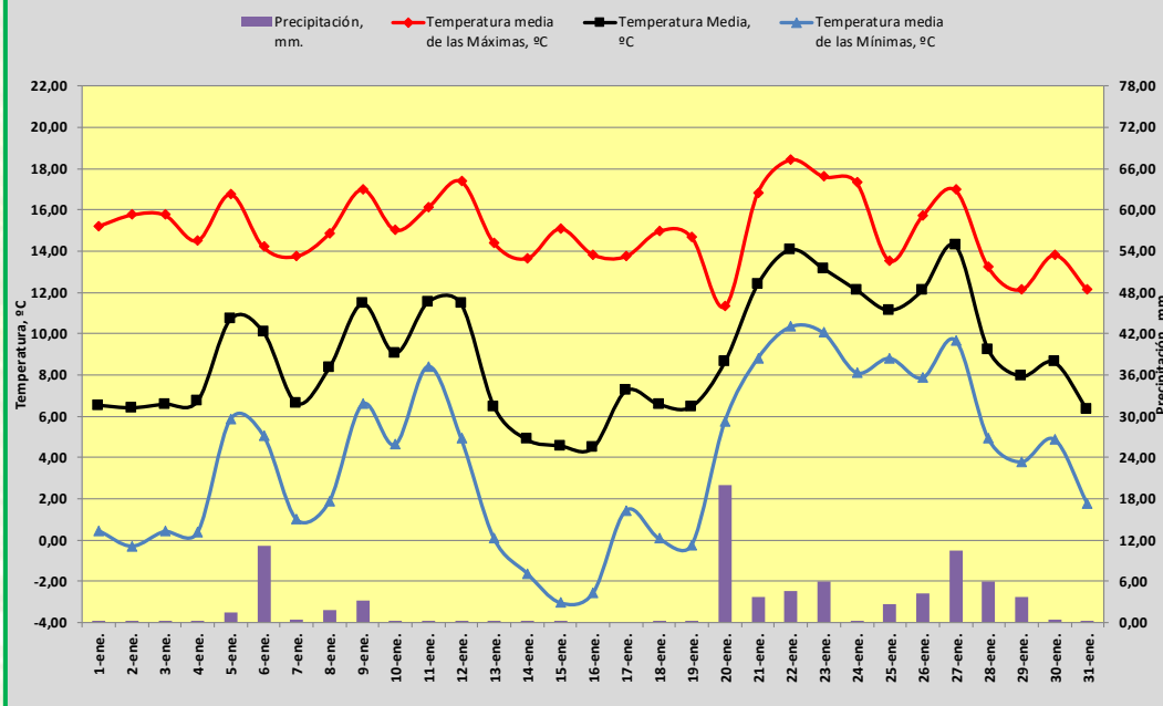
TEMPERATURA Y PRECIPITACIÓN. ENERO DE 2025. CÓRDOBA
