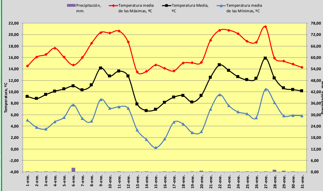
TEMPERATURA Y PRECIPITACIÓN. ENERO DE 2025. ALMERÍA
