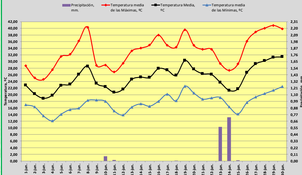
TEMPERATURA Y PRECIPITACIÓN. JUNIO DE 2025. HUELVA
