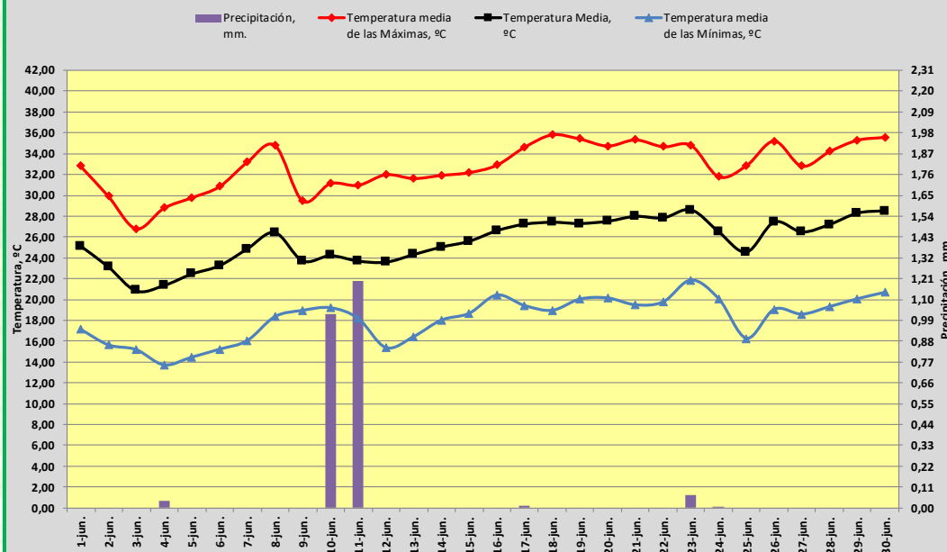
TEMPERATURA Y PRECIPITACIÓN. JUNIO DE 2025. MÁLAGA
