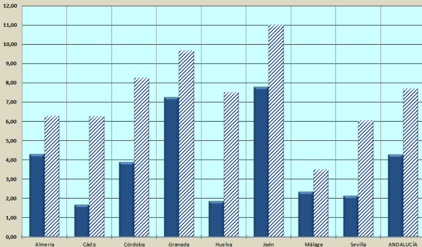
LLUVIA mm. JUNIO.
