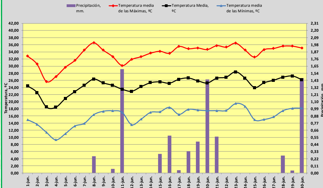
TEMPERATURA Y PRECIPITACIÓN. JUNIO DE 2025. GRANADA
