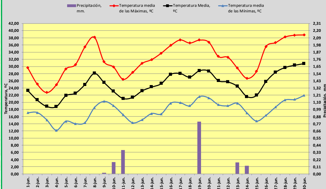
TEMPERATURA Y PRECIPITACIÓN. JUNIO DE 2025. CÁDIZ
