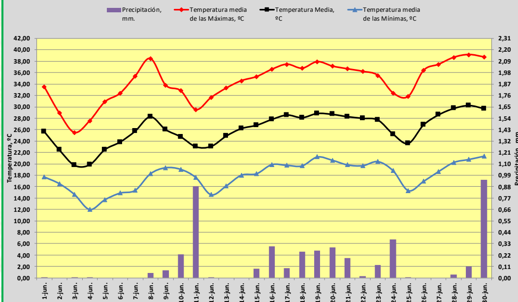
TEMPERATURA Y PRECIPITACIÓN. JUNIO DE 2025. ANDALUCÍA
