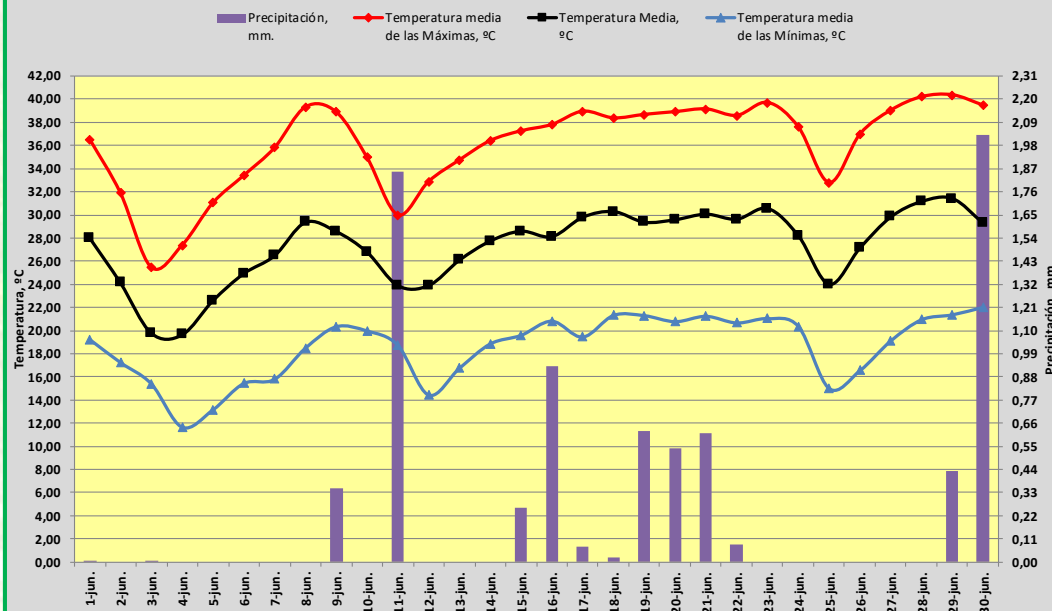
TEMPERATURA Y PRECIPITACIÓN. JUNIO DE 2025. JAÉN
