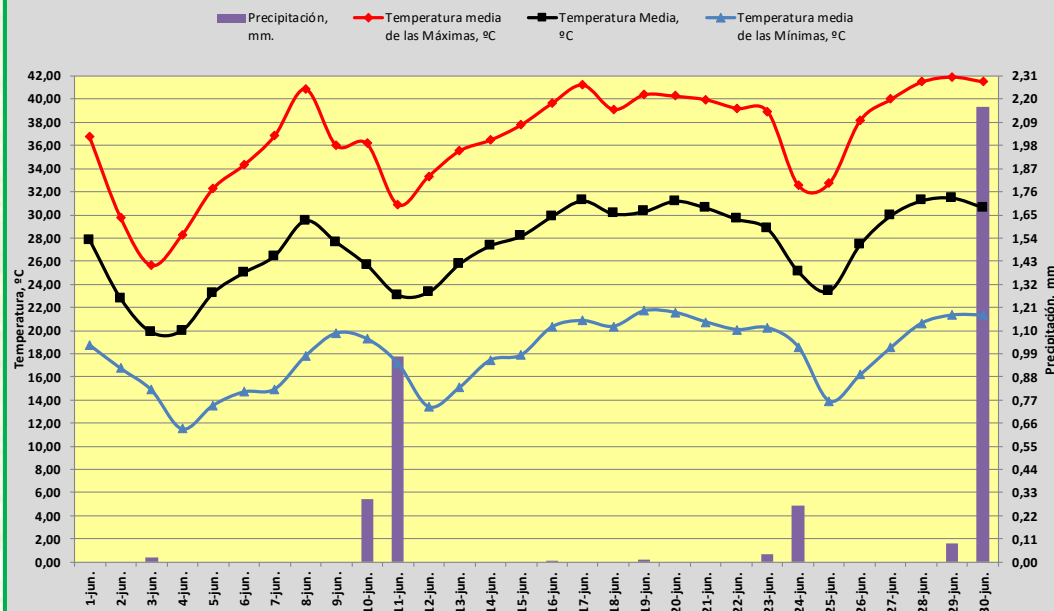
TEMPERATURA Y PRECIPITACIÓN. JUNIO DE 2025. CÓRDOBA
