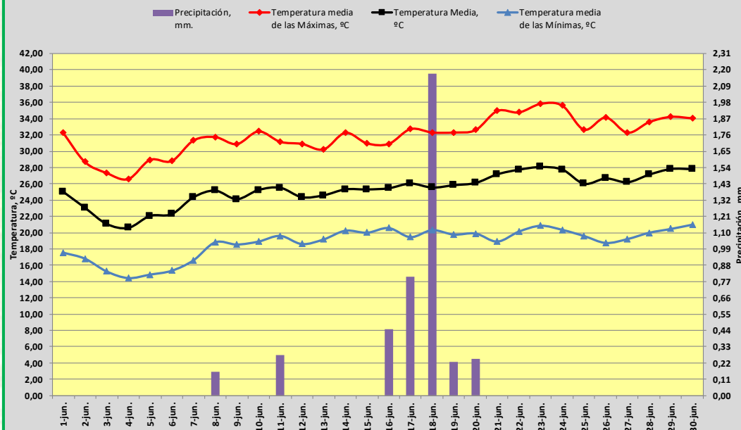
TEMPERATURA Y PRECIPITACIÓN. JUNIO DE 2025. ALMERÍA
