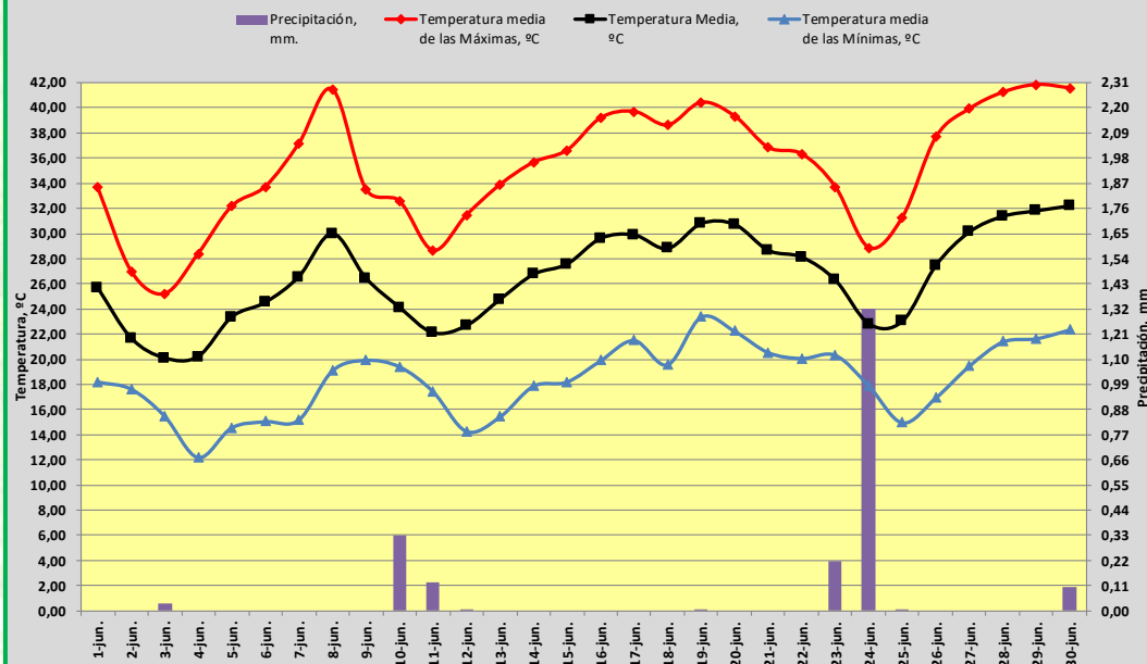
TEMPERATURA Y PRECIPITACIÓN. JUNIO DE 2025. SEVILLA
