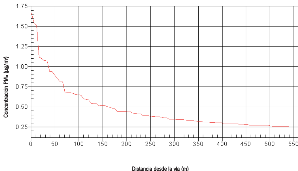
Figura 7.6 Evolución de la concentración de PM 10 con la distancia. Avenida Montes Sierra
