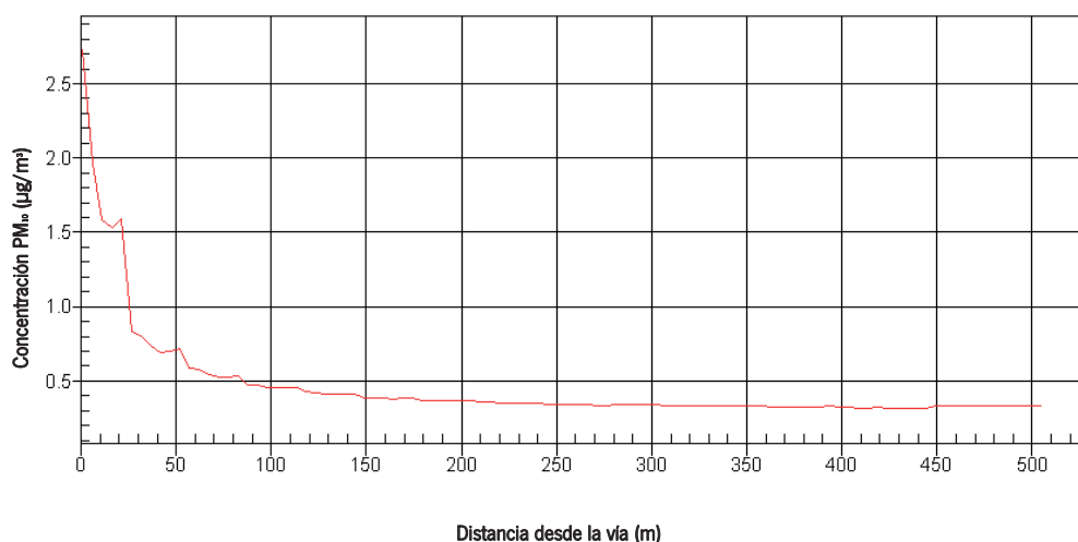
Figura 7.8 Evolución de la concentración de PM 10 con la distancia. Avenida de la Palmera
