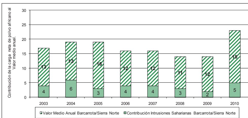
Figura 5.17 Contribución de la carga neta de polvo africano al valor medio anual en las estaciones de fondo-regional Barcarrota (2003-2009) y la estación de fondo-rural Sierra Norte (2010).
