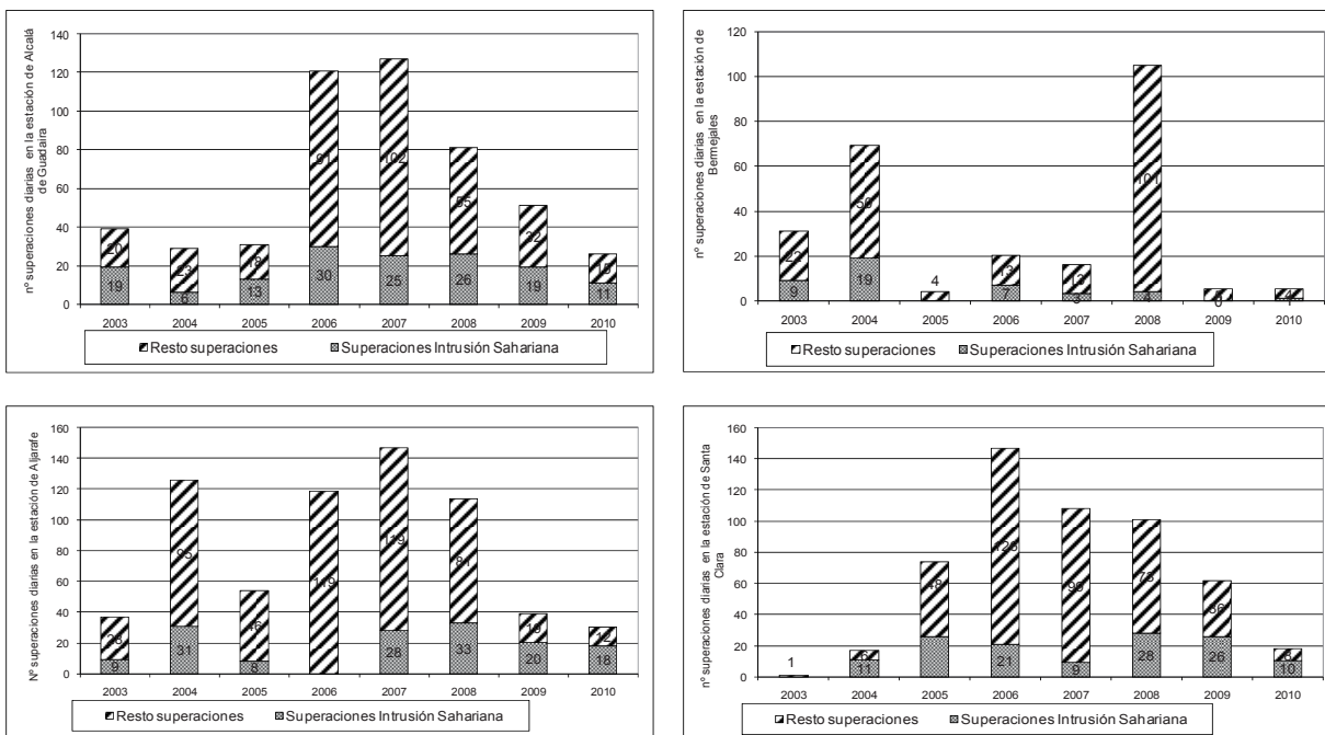
Figura 5.13 Origen y cuantificación del número de superaciones diarias de PM 10 (µg/m 3 ) en las estaciones de Alcalá de Guadaíra, Aljarafe, Bermejales y Santa Clara
