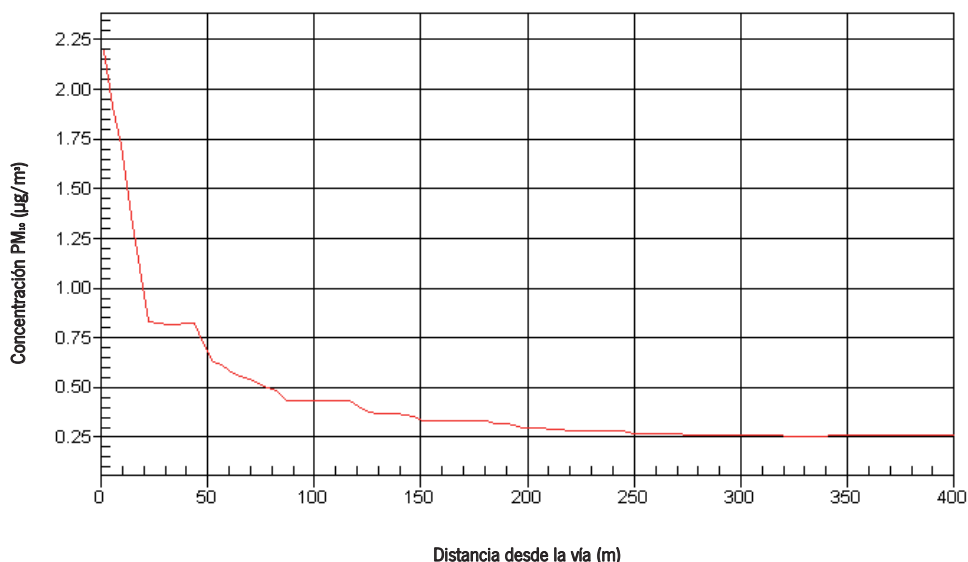
Figura 7.10 Evolución de la concentración de PM 10 con la distancia. Avenida del 28 de Febrero
