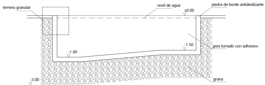
Sección constructiva
