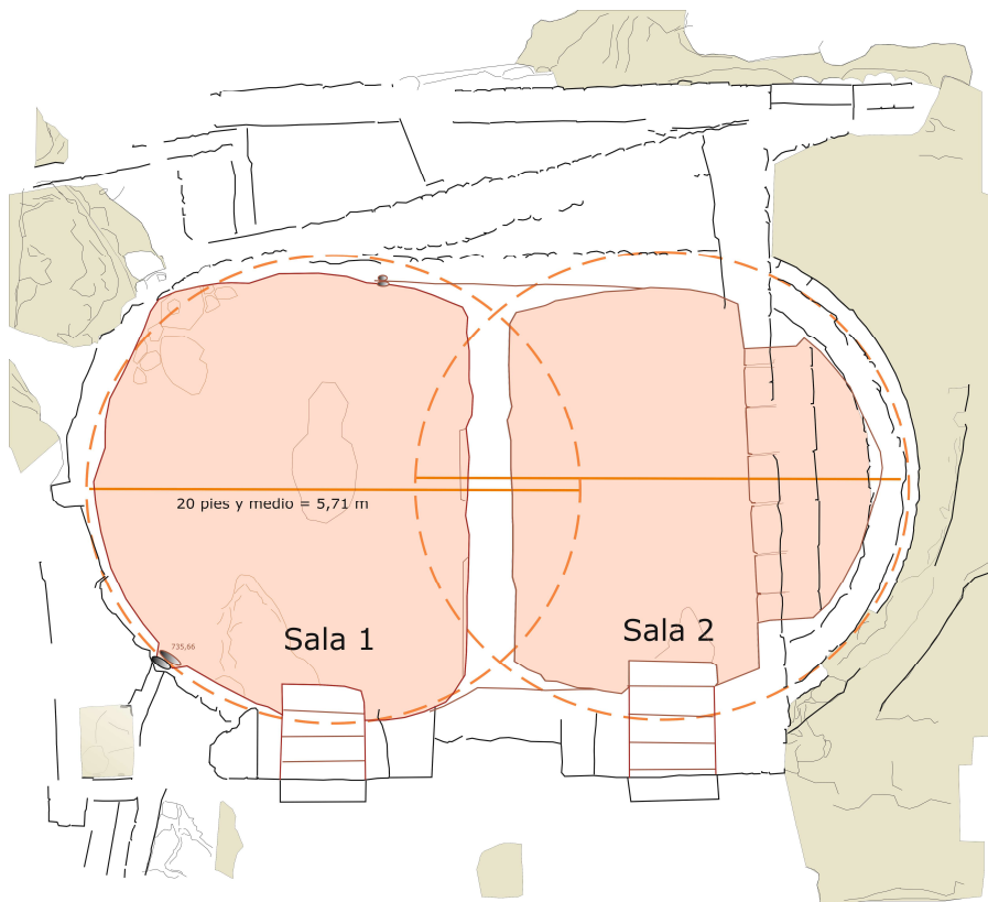
Figura 9: Planta de los baños con la geometría utilizada en su construcción.
