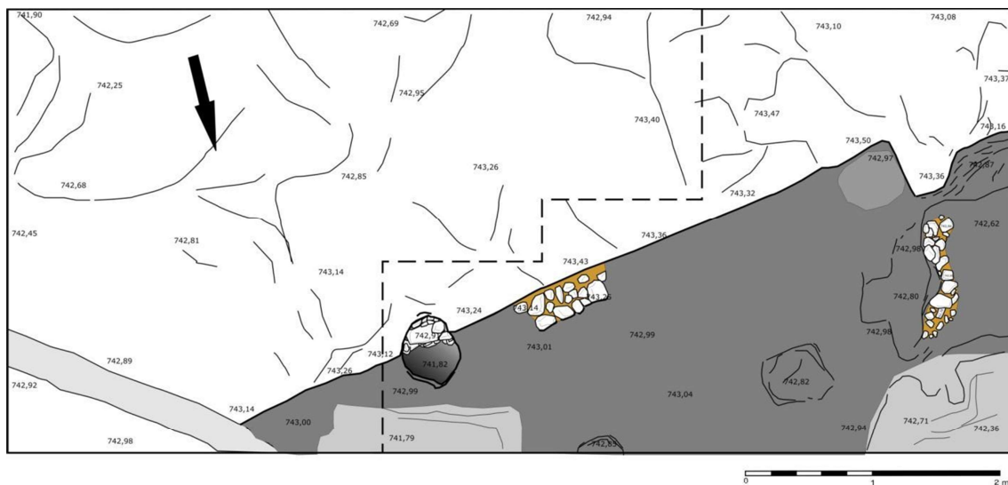
Figura 5: Planta final del Corte 14, en gris oscuro el rebaje del terreno para la ubicación del almacén y el silo.
