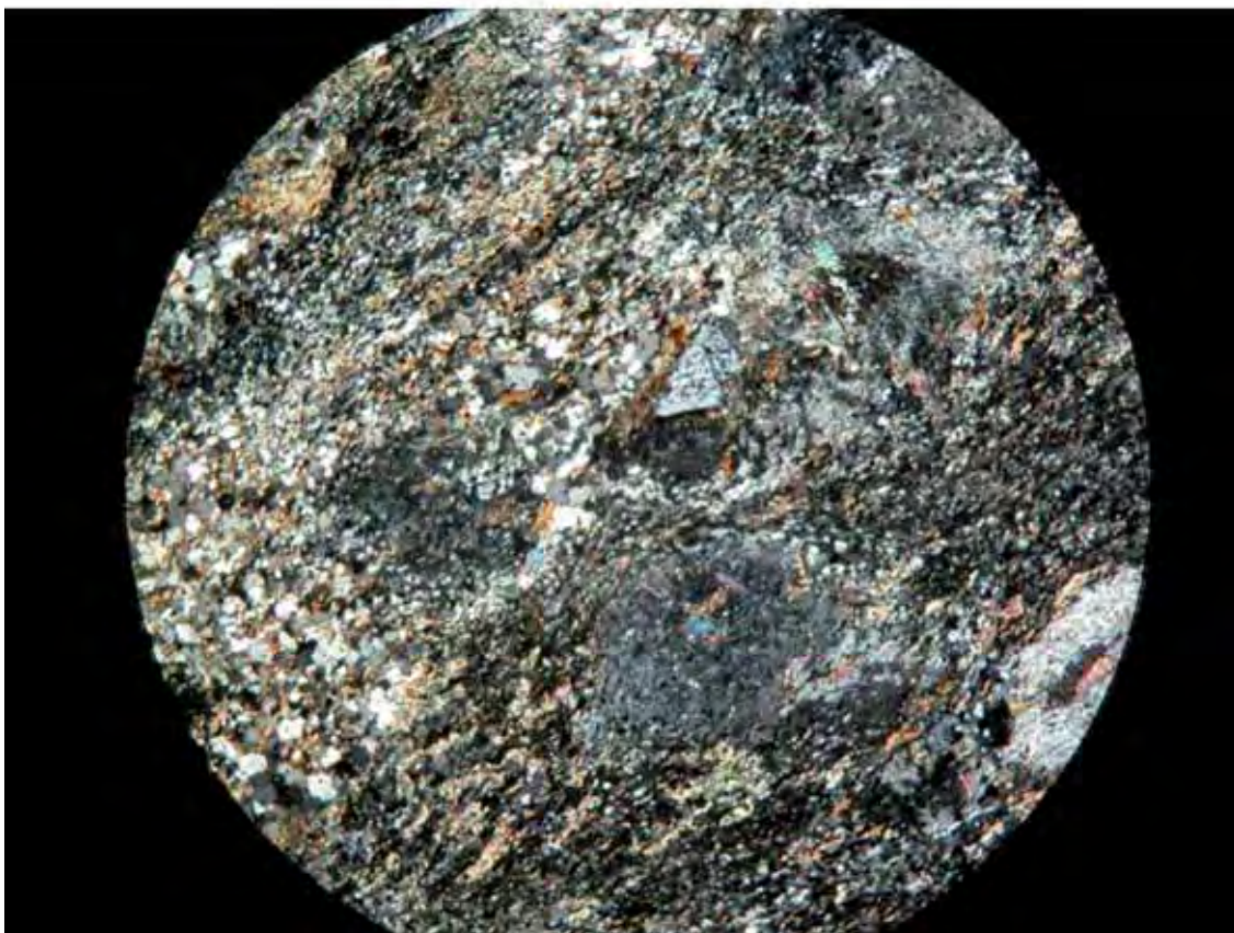
Lámina 7.6. Esquisto moteado con andalucita. Zona de Ossa-Morena, Macizo Hercínico. Foto superior con nicoles paralelos e inferior con nicoles cruzados. El ancho de la foto corresponde aproximadamente a 1 mm.
