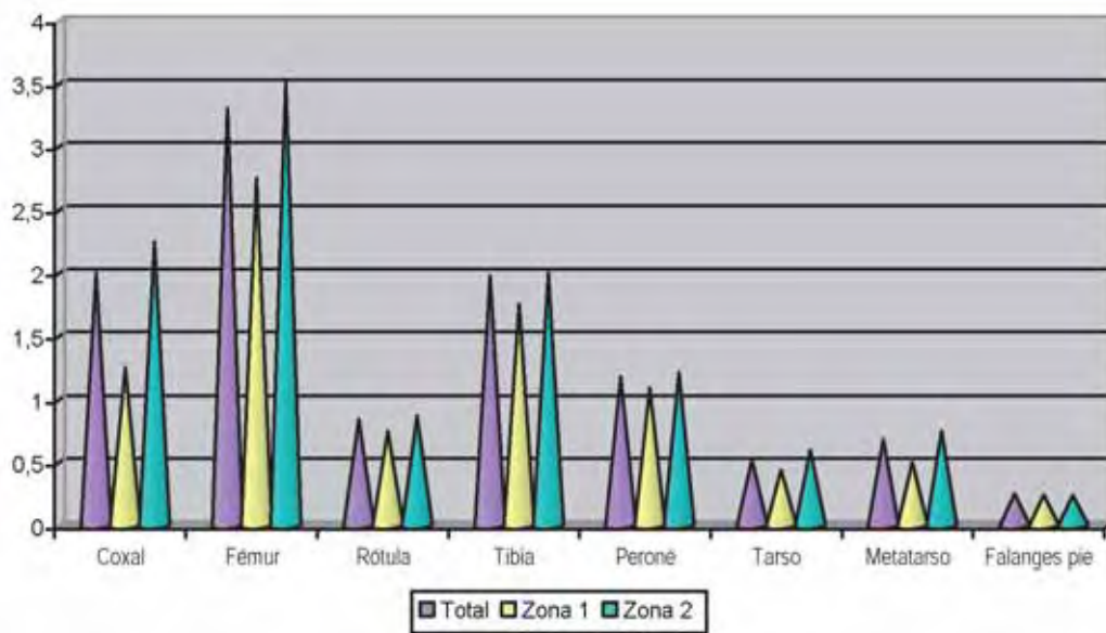
Figura 6.36. Relación de elementos óseos de la extremidad inferior identificados y elementos óseos esperados según el mínimo número de individuos
