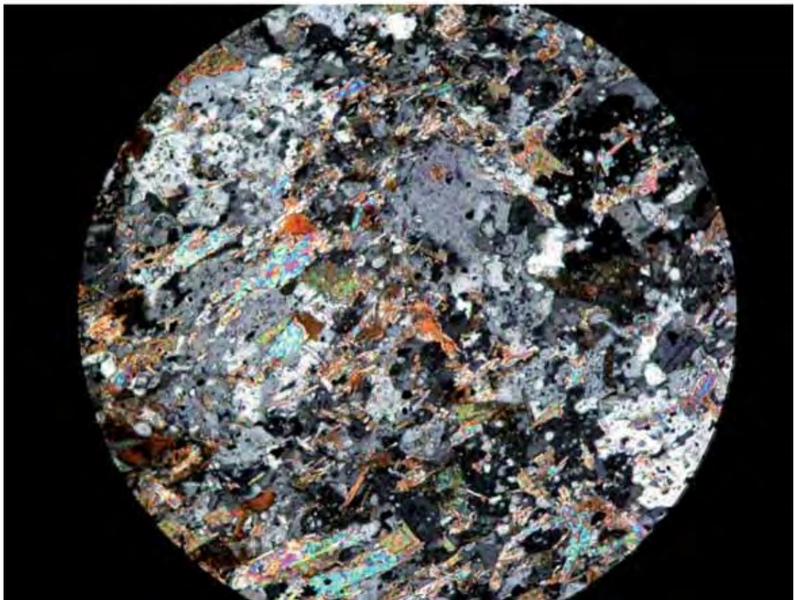
Lámina 7.5. Esquisto con epidota. Zona de Ossa-Morena, Macizo Hercínico. Foto superior con nícoles paralelos e inferior con nícoles cruzados. El ancho de la foto corresponde aproximadamente a 1 mm.
