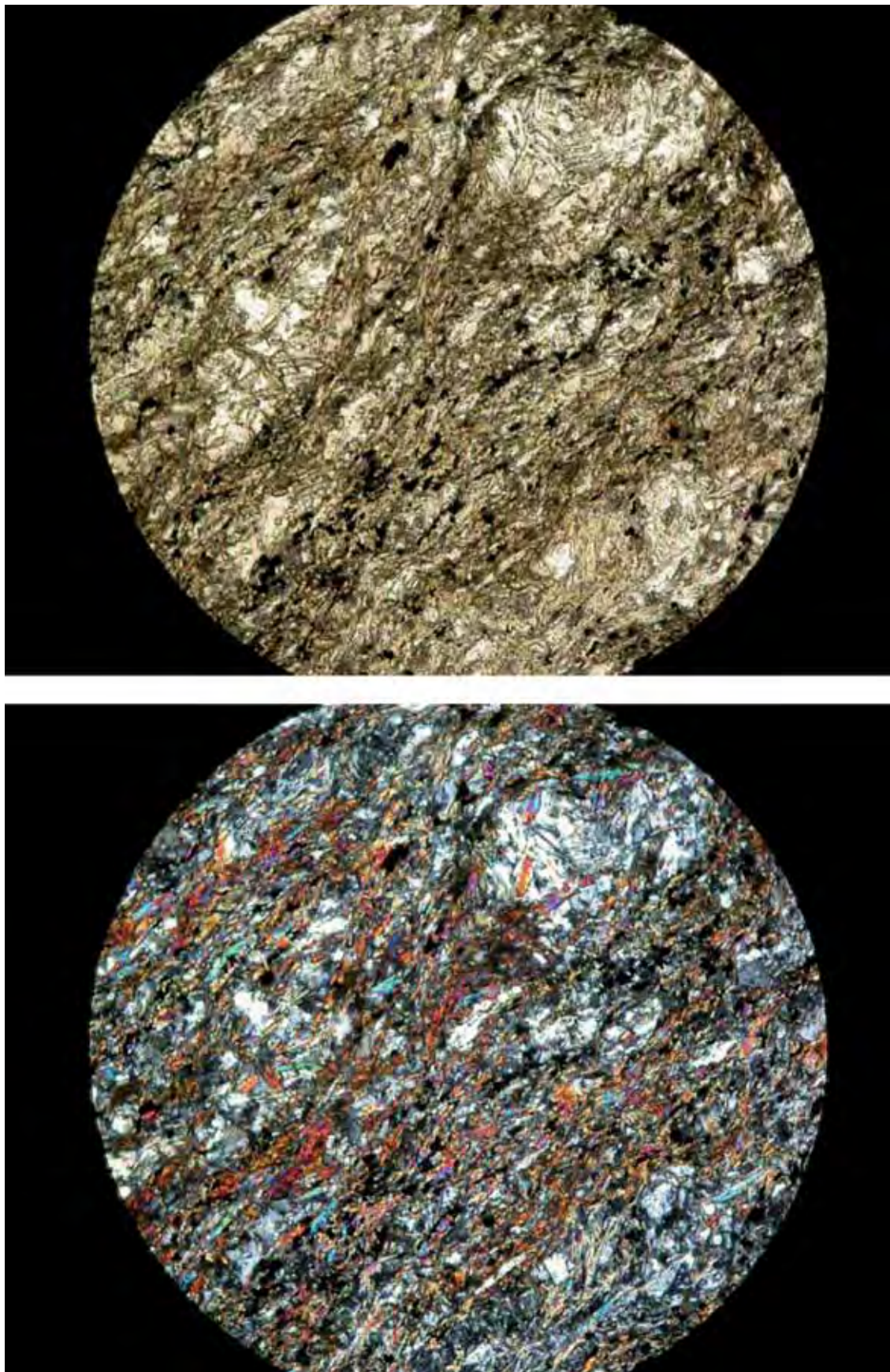
Lámina 7.4. Anfibolita. Zona de Ossa-Morena, Macizo Hercínico. Foto superior con nícoles paralelos e inferior con nícoles cruzados. El ancho de la foto corresponde aproximadamente a 1 mm.
