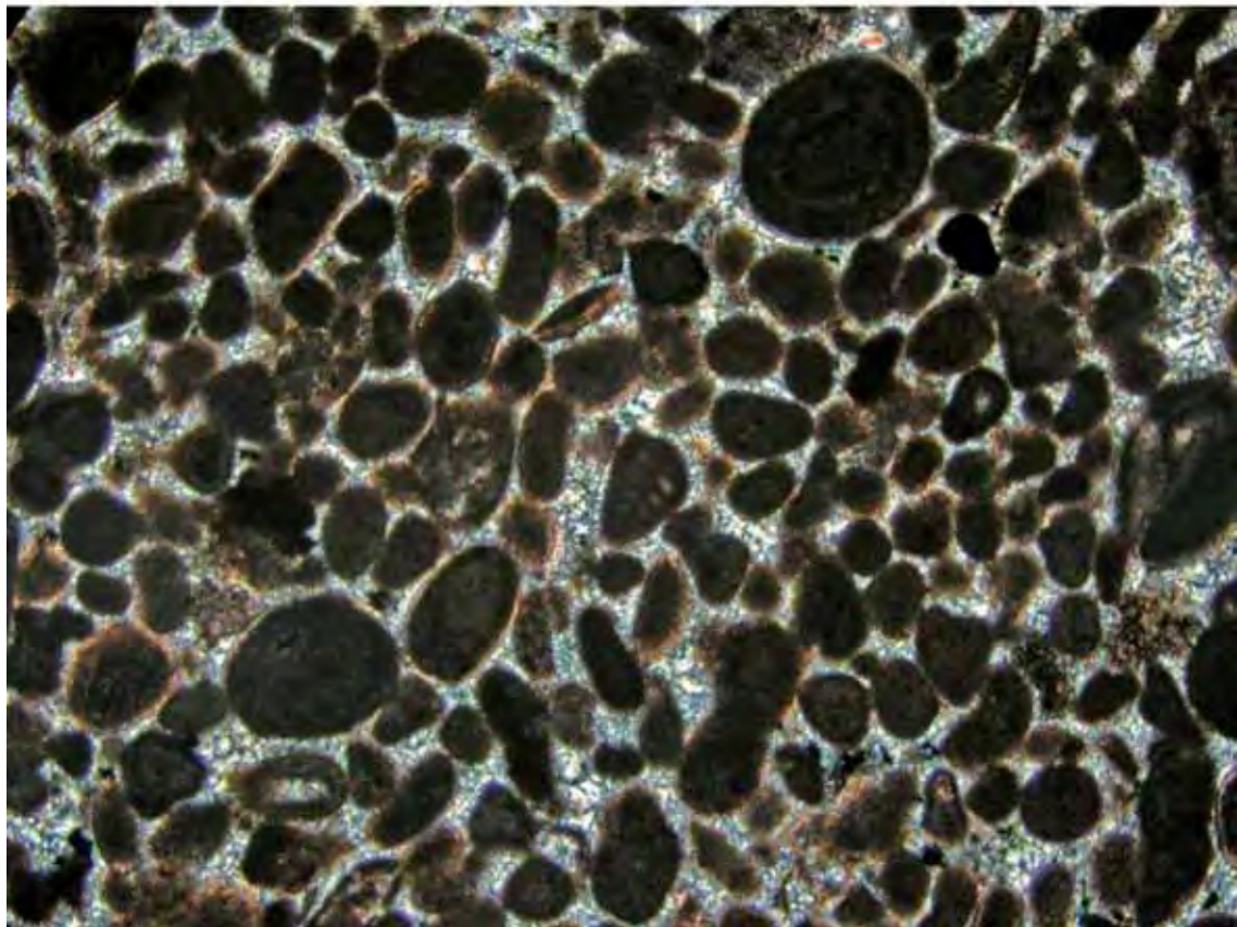
Lámina 7.1. Caliza oolítica parcialmente silicificada (matriz). Zonas Externas de las Cordilleras Béticas. Foto superior con nícoles paralelos e inferior con nícoles cruzados. El ancho de la foto corresponde aproximadamente a 1 mm.
