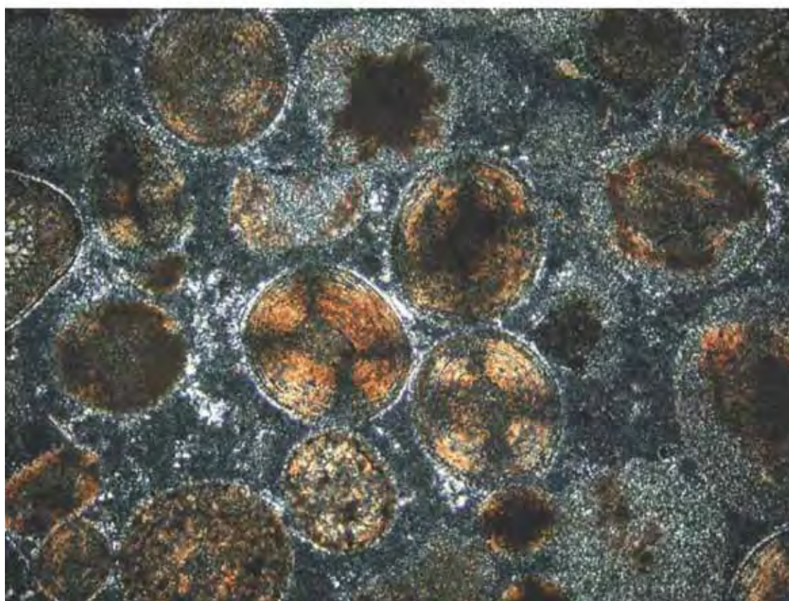
Lámina 7.2. Caliza oolítica parcialmente silicificada (matriz y parte externa de los oolitos). Zonas Externas de las Cordilleras Béticas. Foto superior con nícoles paralelos e inferior con nícoles cruzados. El ancho de la foto corresponde aproximadamente a 1 mm.
