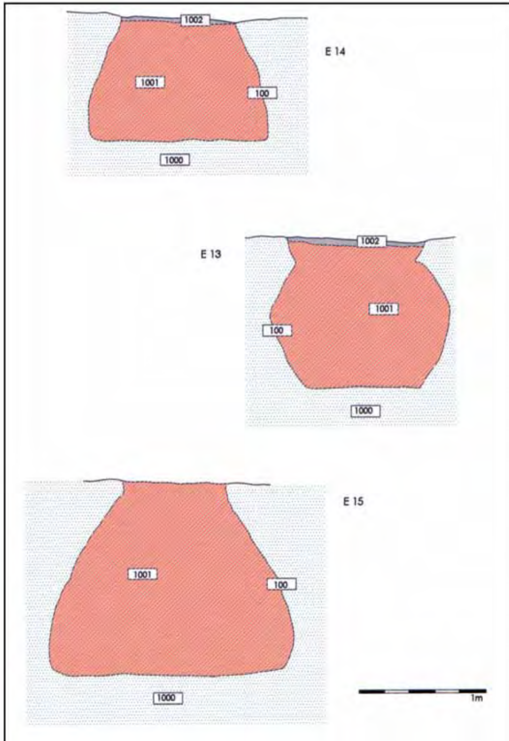
Figura 3.2. Perfiles silos
