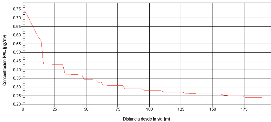
Figura 7.2 Evolución de la concentración de PM 10 con la distancia. Carretera Nacional 340a
