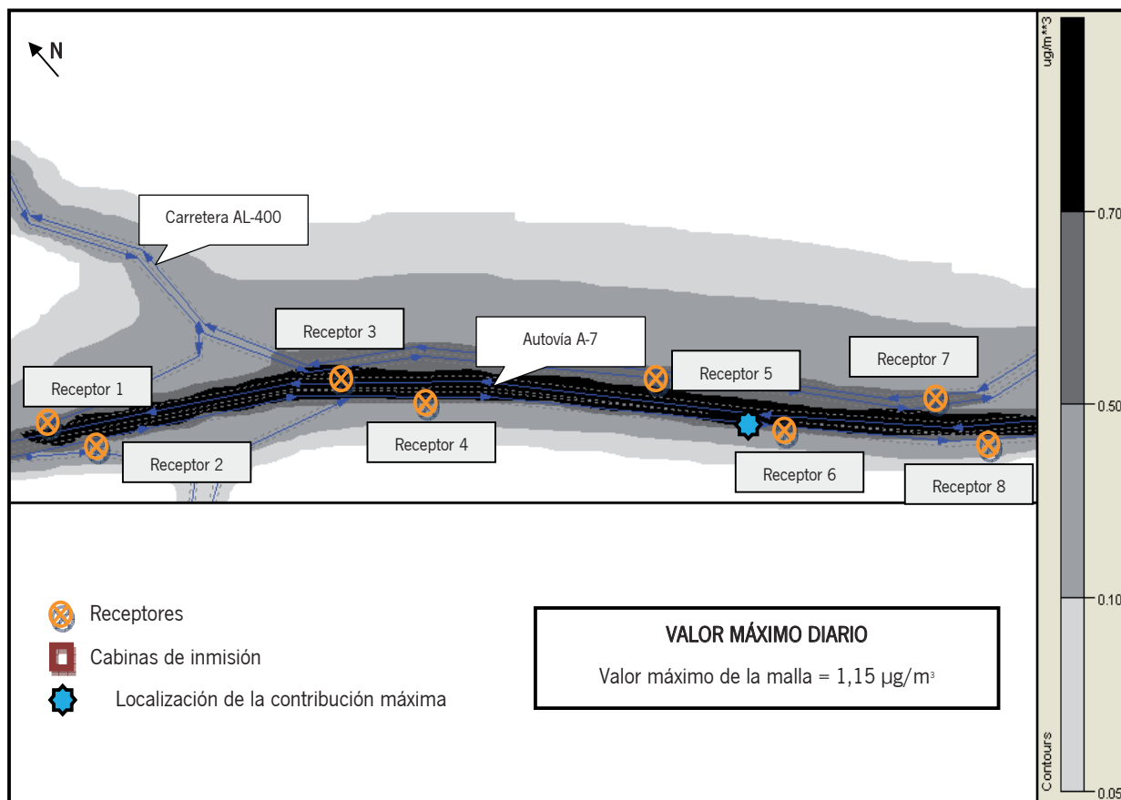
Figura 7.3 Contribución del tráfico en El Ejido a la media anual de PM 10 . Autovía A-7
