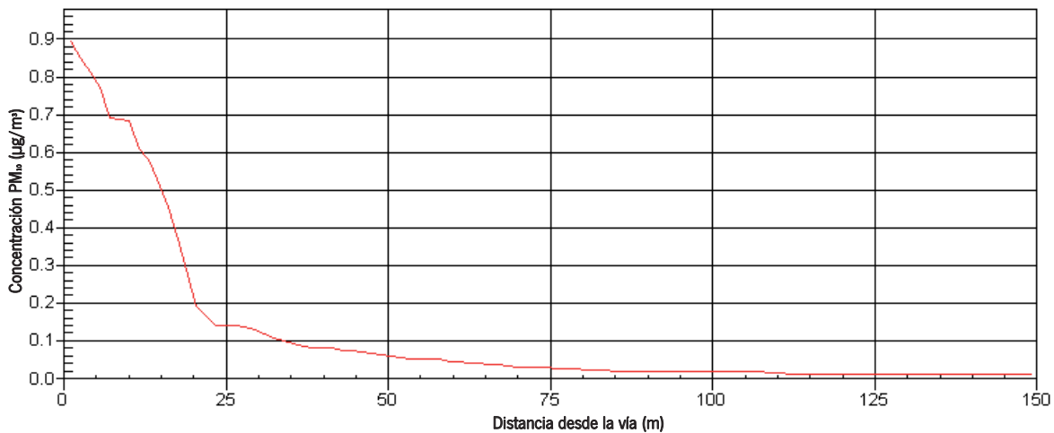
Figura 7.4 Evolución de la concentración de PM_{10} con la distancia. Autovía A-7
