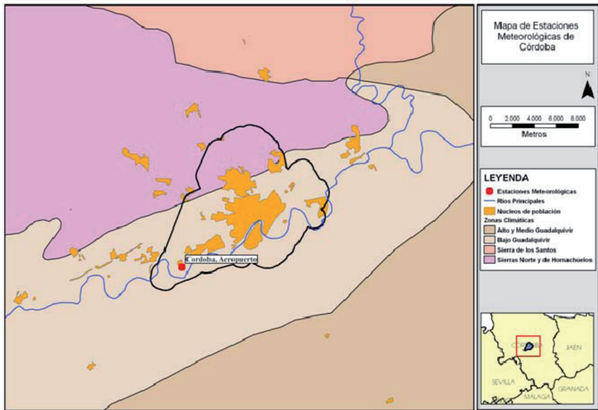
Figura 4.4. Análisis climatológico.
