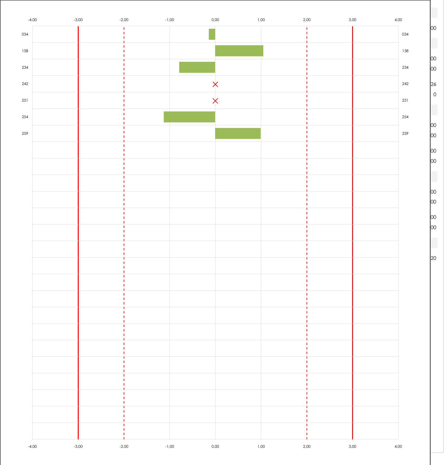
Laboratorio (--- ; eje Y) vs valores Z-Score "prof.maxim.penet.agua hormigon" (--- ; eje X)
