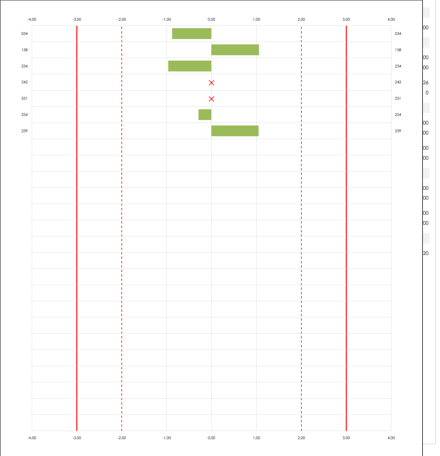
Laboratorio (--- ; eje Y) vs valores Z-Score "prof.media.penet.agua hormigon" (--- ; eje X)
