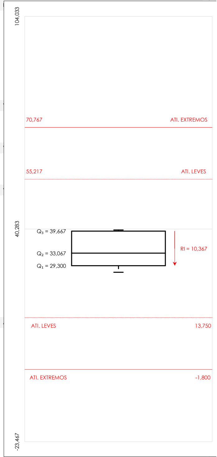
Diagrama Box-Plot post-estadístico. Eje Y: prof.maxim.penet.agua hormigon (mm)
