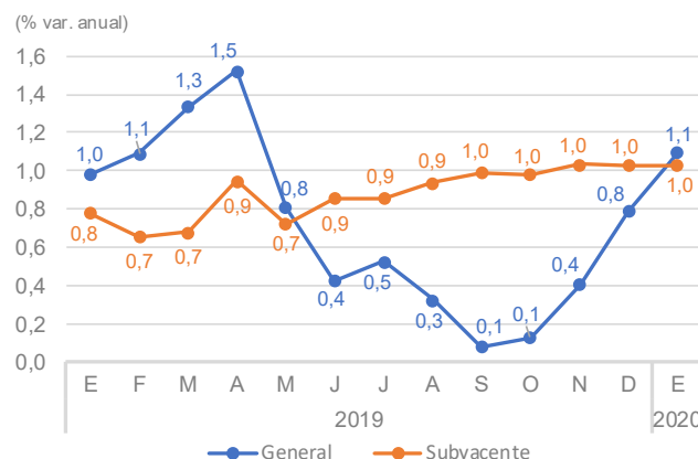
Gráfico 5. IPC. España
