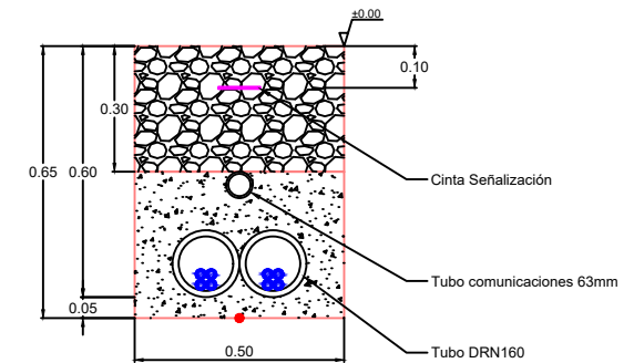
TIPO BT-II-H Canalización de 2 circuitos AC
