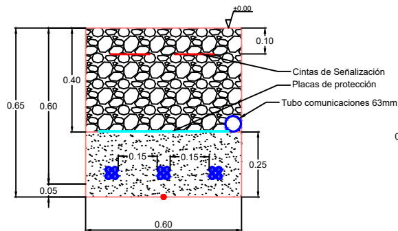
TIPO BT-III Canalización de 3 circuitos AC
