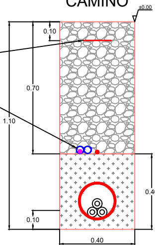
TIPO MV-II 1 circuito MT CAMINO
