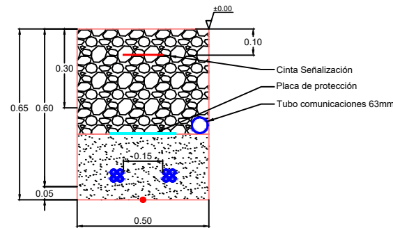
TIPO BT-II Canalización de 2 circuitos AC
