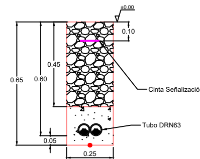
TIPO DC Canalización De 1-10 Strings DC
