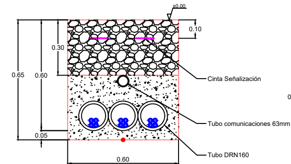
TIPO BT-III-H Canalización de 3 circuitos AC
