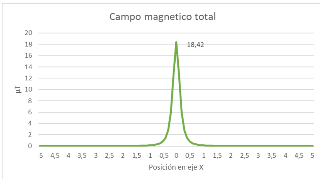
Ilustración 8: Campo magnético a 200 mm del borde del cable
