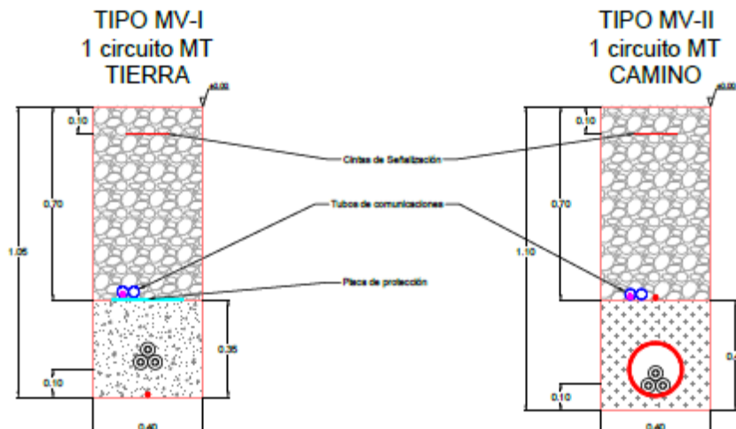
Ilustración 12:Detalle de zanjas MT normal y reforzada
