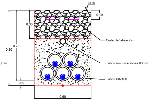
TIPO BT-IV-H Canalización de 4-5 circuitos AC
