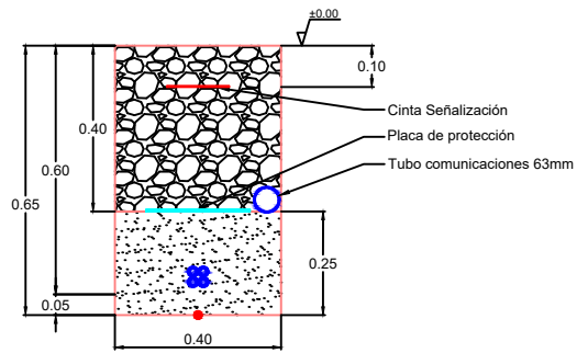
TIPO BT-I Canalización de 1 circuito AC
