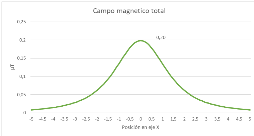
Ilustración 7: Campo magnético a 1 metro de altura respecto al terreno
