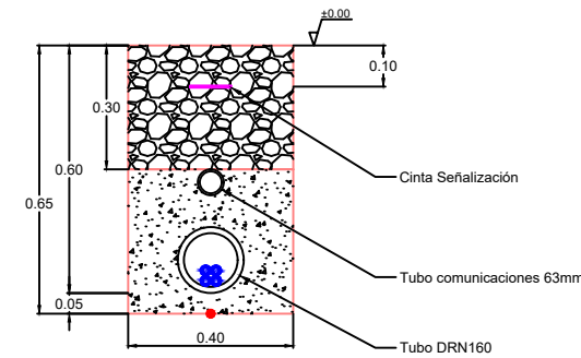
TIPO BT-I-H Canalización de 1 circuito AC
