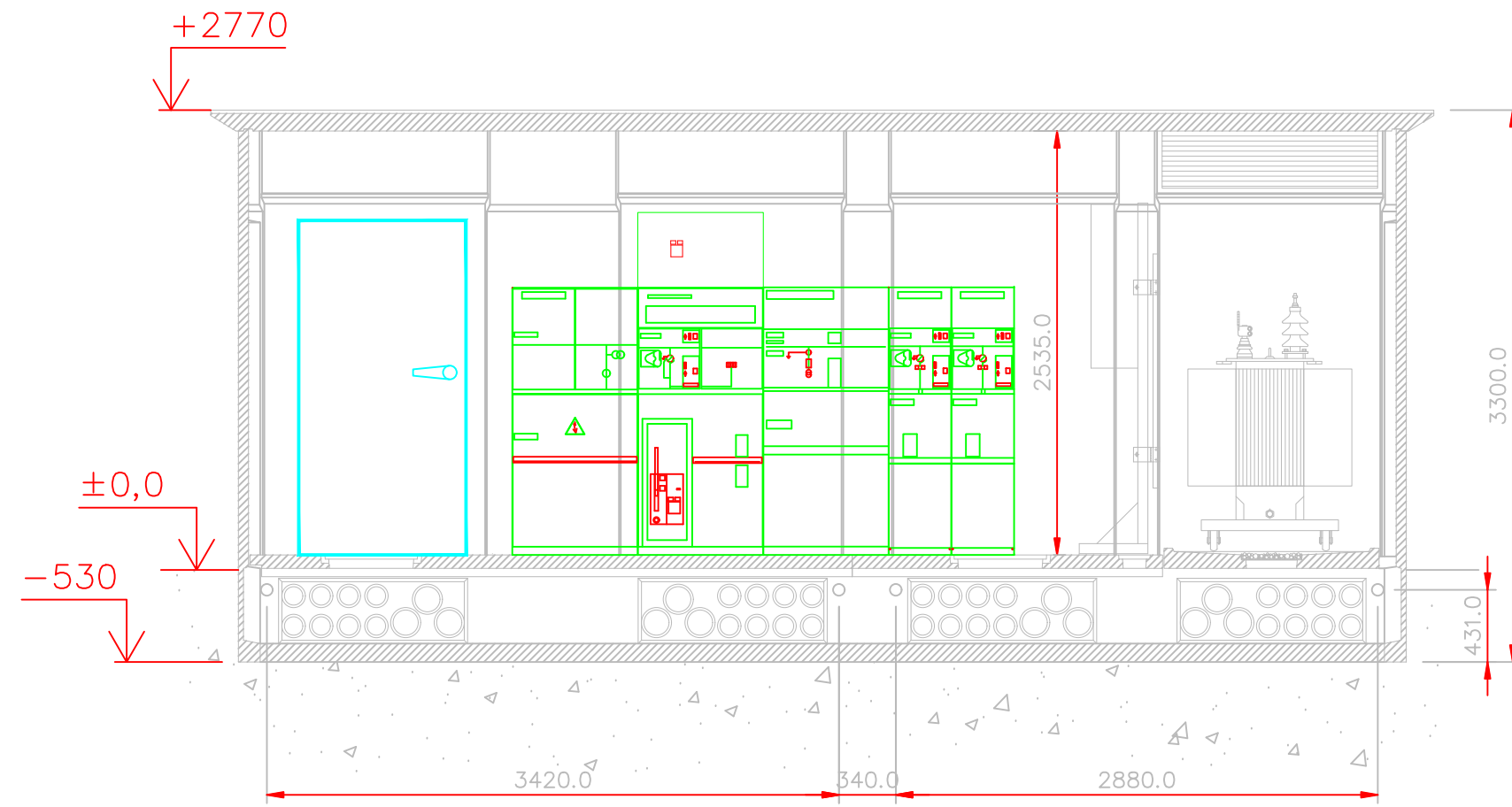
SECCIÓN
