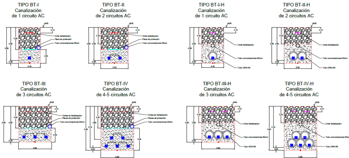
Ilustración 11: Detalle de zanjas BT normal y reforzada hasta 5 circuitos
