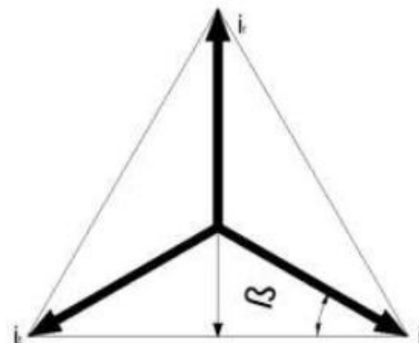
Ilustración 6: Circuito trifásico equilibrado
