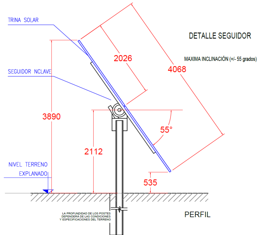
Ilustración 9: Detalle altura máxima de seguidor
