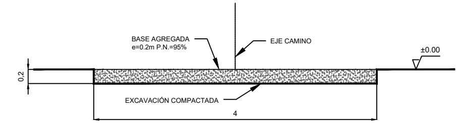
DETALLE CAMINO INTERIOR
