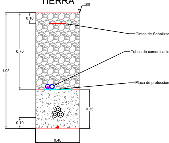
TIPO MV-I 1 circuito MT TIERRA
