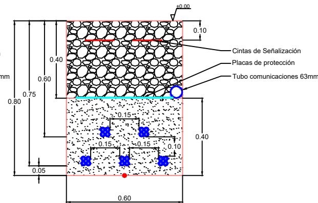
TIPO BT-IV Canalización de 4-5 circuitos AC
