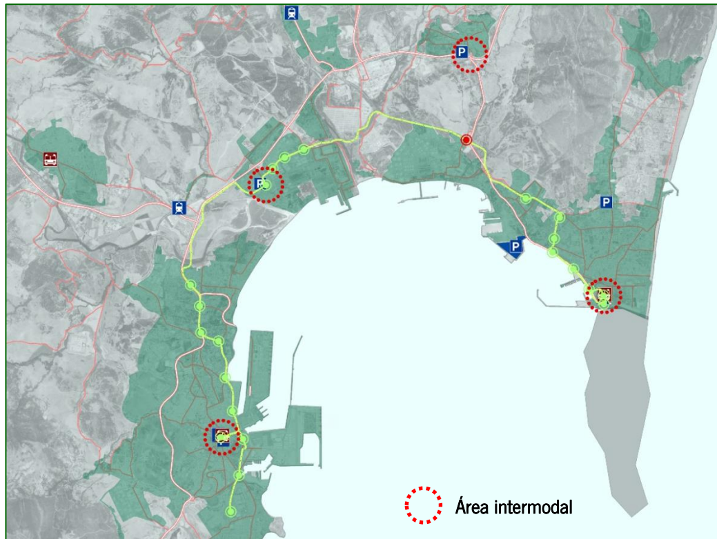
Figura 12.1: Mapa general de las área intermodales propuestas.
