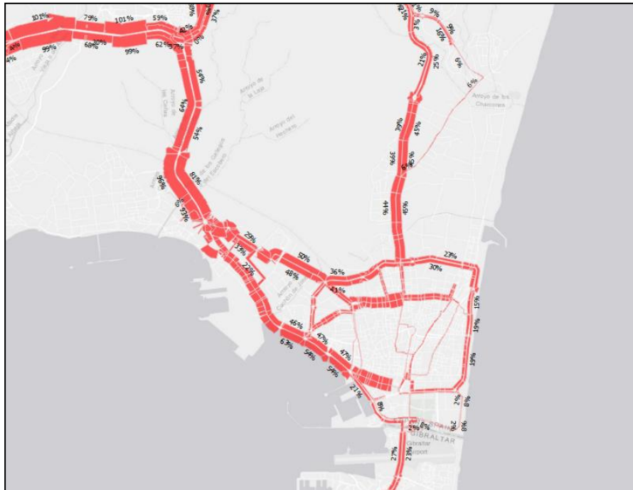
Figura 8.2: Mapa V/C en la CA-34.
