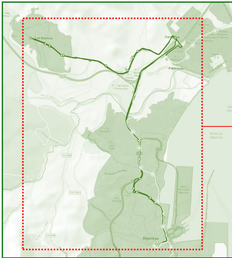
Figura 12.34: Comprobación cobertura por la supresión de las líneas M-112.
