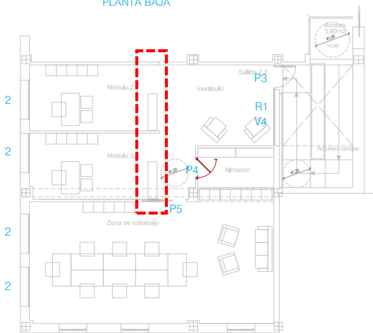
PLANTA BAJA
