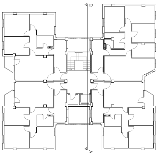
PLANTA DE PISOS
