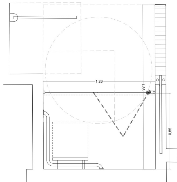
Mampara ducha M1 Frontal de ducha de vidrio templado de 6mm. Apertura plegable, bisagras de aluminio. Tirador de doble asa. Cierre imantado.
