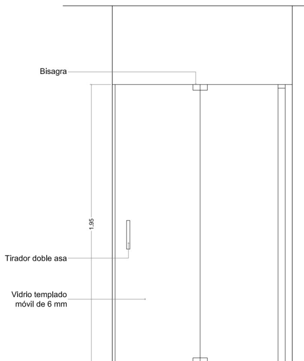
Mampara ducha M1 Frontal de ducha de vidrio templado de 6mm. Apertura plegable, bisagras de aluminio. Tirador de doble asa. Cierre imantado.
