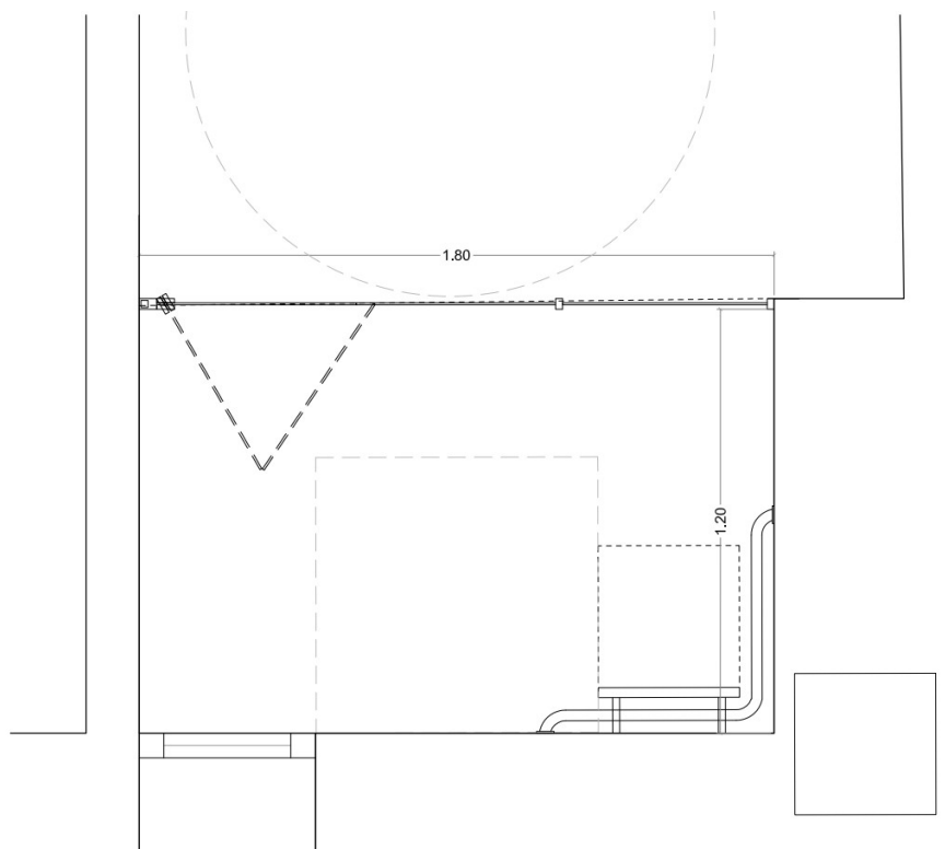
Mampara ducha M4 Frontal de ducha de vidrio templado de 6mm (1 fijo + 2 plegables). Apertura plegable. Tirador de doble asa. Cierre imantado.
