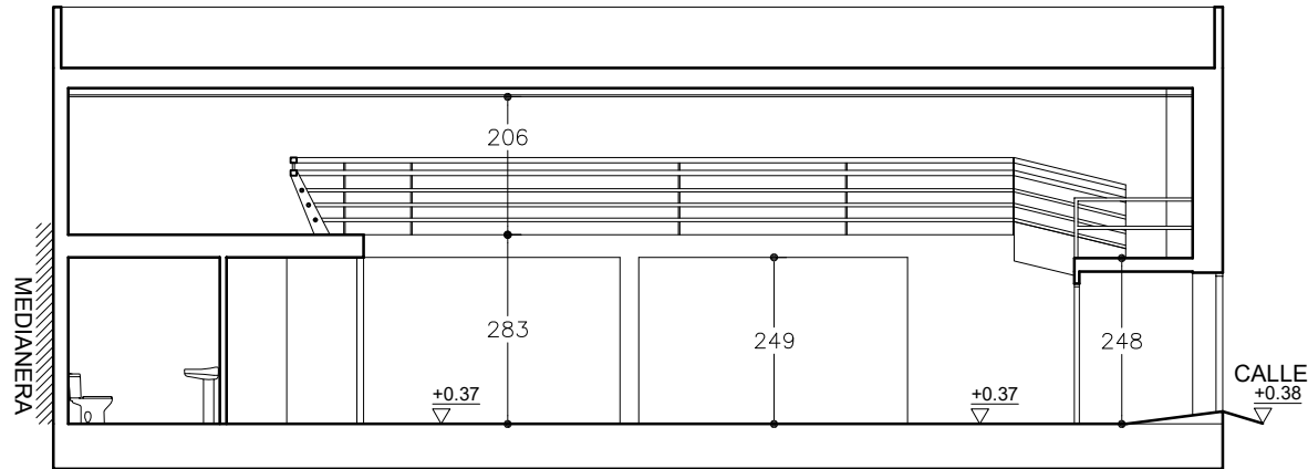
SECCIÓN TRANSVERSAL 4
