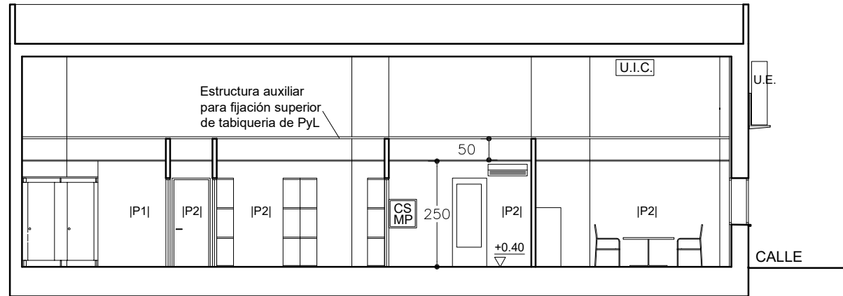
SECCIÓN TRANSVERSAL 4
