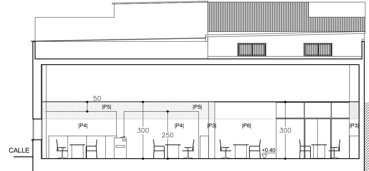
SECCIÓN TRANSVERSAL 2
