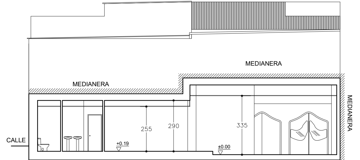
SECCIÓN TRANSVERSAL 1
