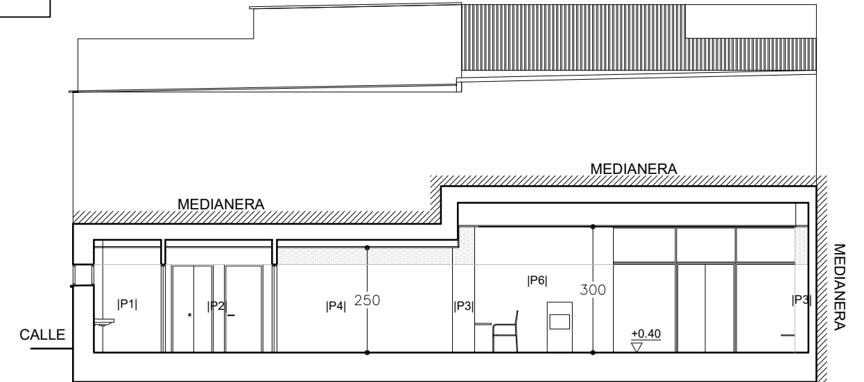
SECCIÓN TRANSVERSAL 1
