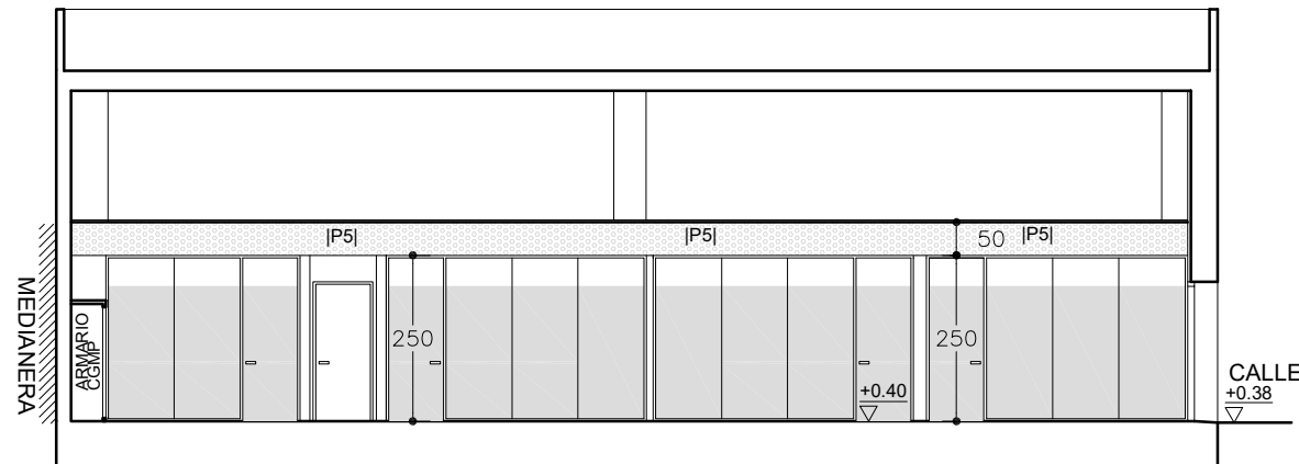
SECCIÓN TRANSVERSAL 3
