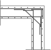
Detalle Esquina Muro Foso
