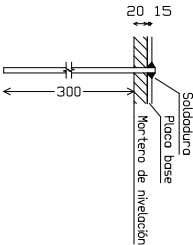
Detalle Anclaje Perno
