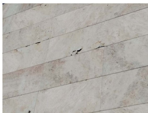
Deterioro generalizado en piezas de aplacado.
