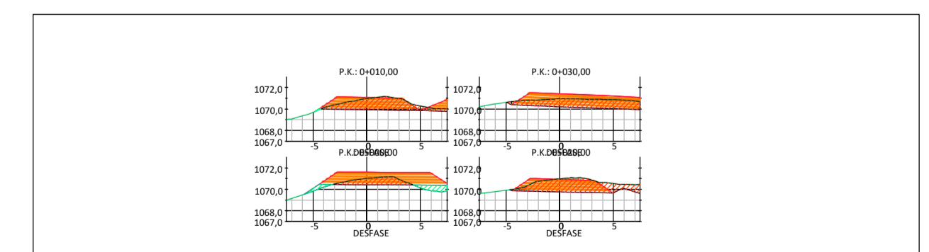
Carril de cambio de sentido. Escala 1 : 500
