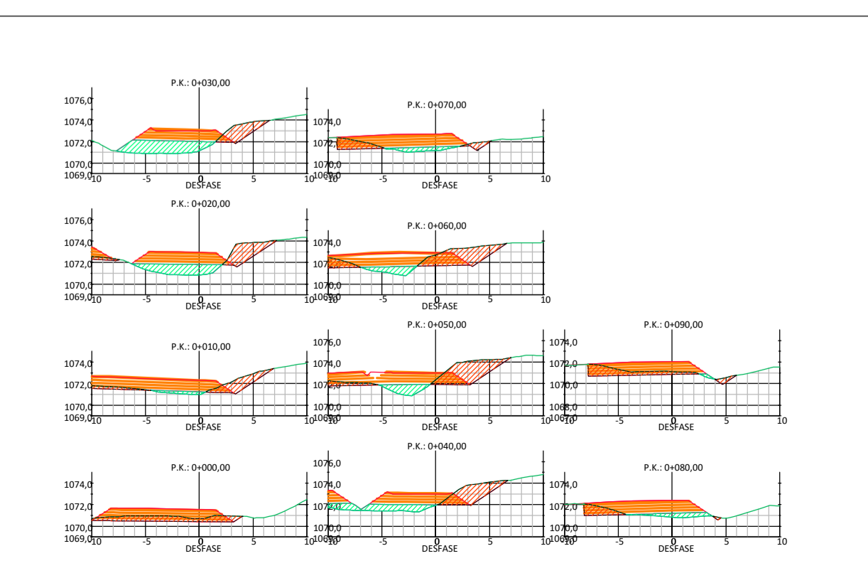
Carril de aceleración. Escala 1 : 500
