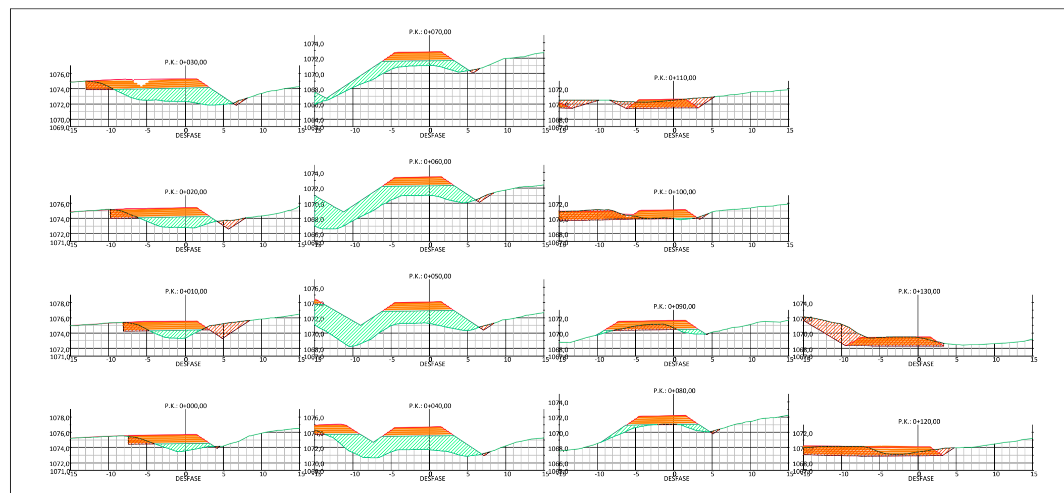
Carril de deceleración. Escala 1 : 500
