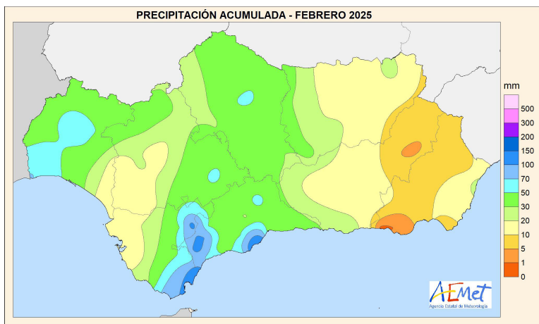
Precipitación mensual
