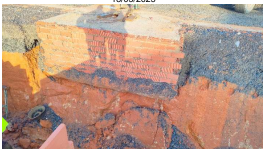
Desprendimiento de tierras en cimentaciones
