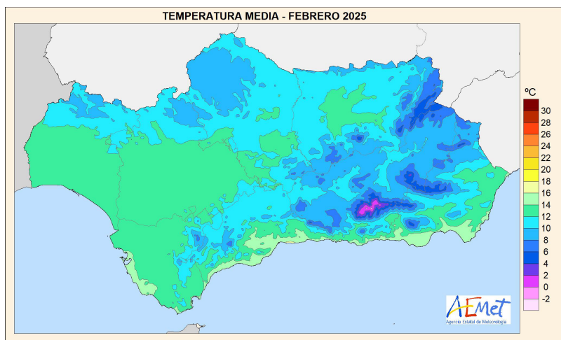
Temperatura media
