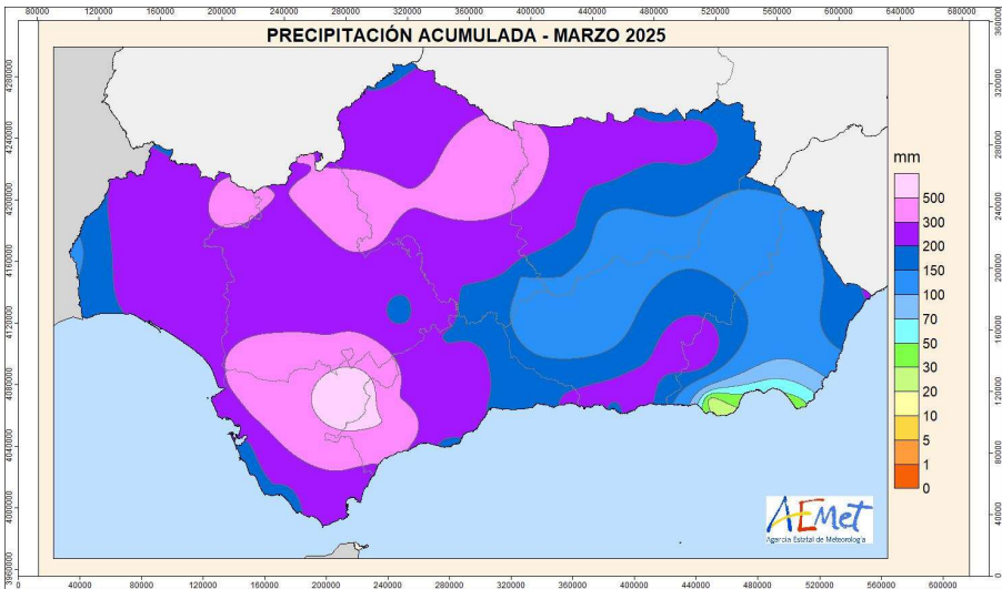
Precipitación mensual
