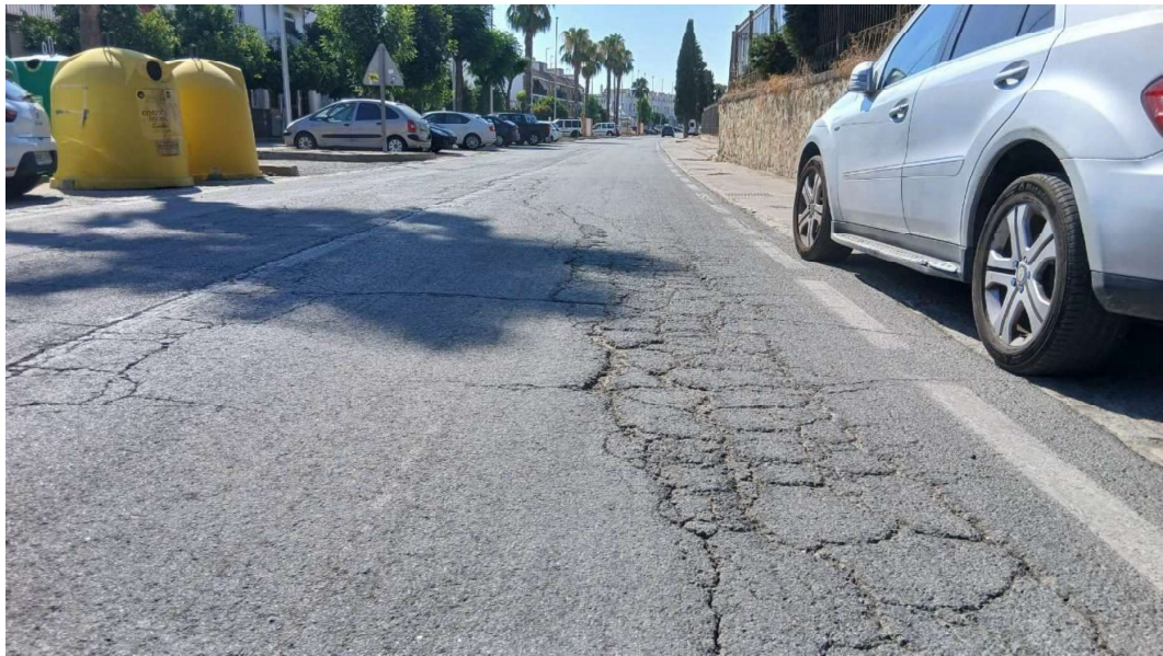
Foto N° 7: Fotos del estado del firme en la A-8078 p.k. 3+500 al 4+200
