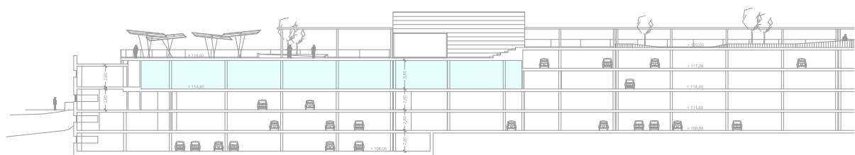
SECCION LONGITUDINAL A-A'
