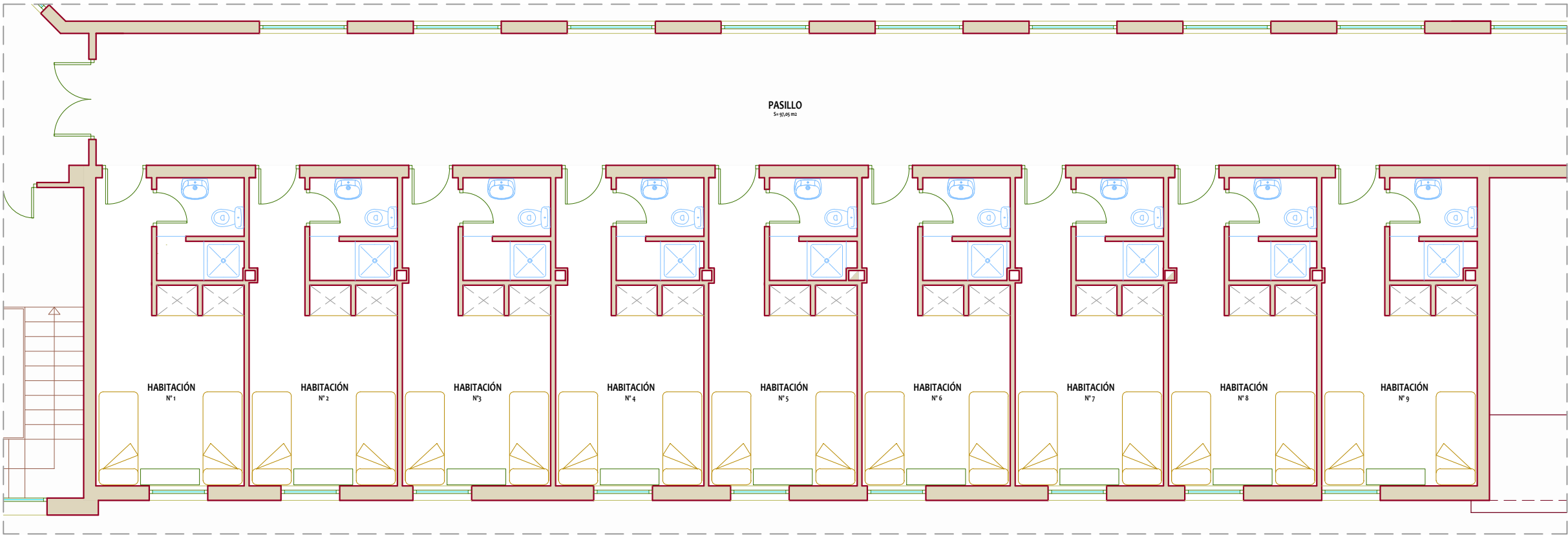
ALA DERECHA PLANTA SEGUNDA. ESTADO ACTUAL BA3
