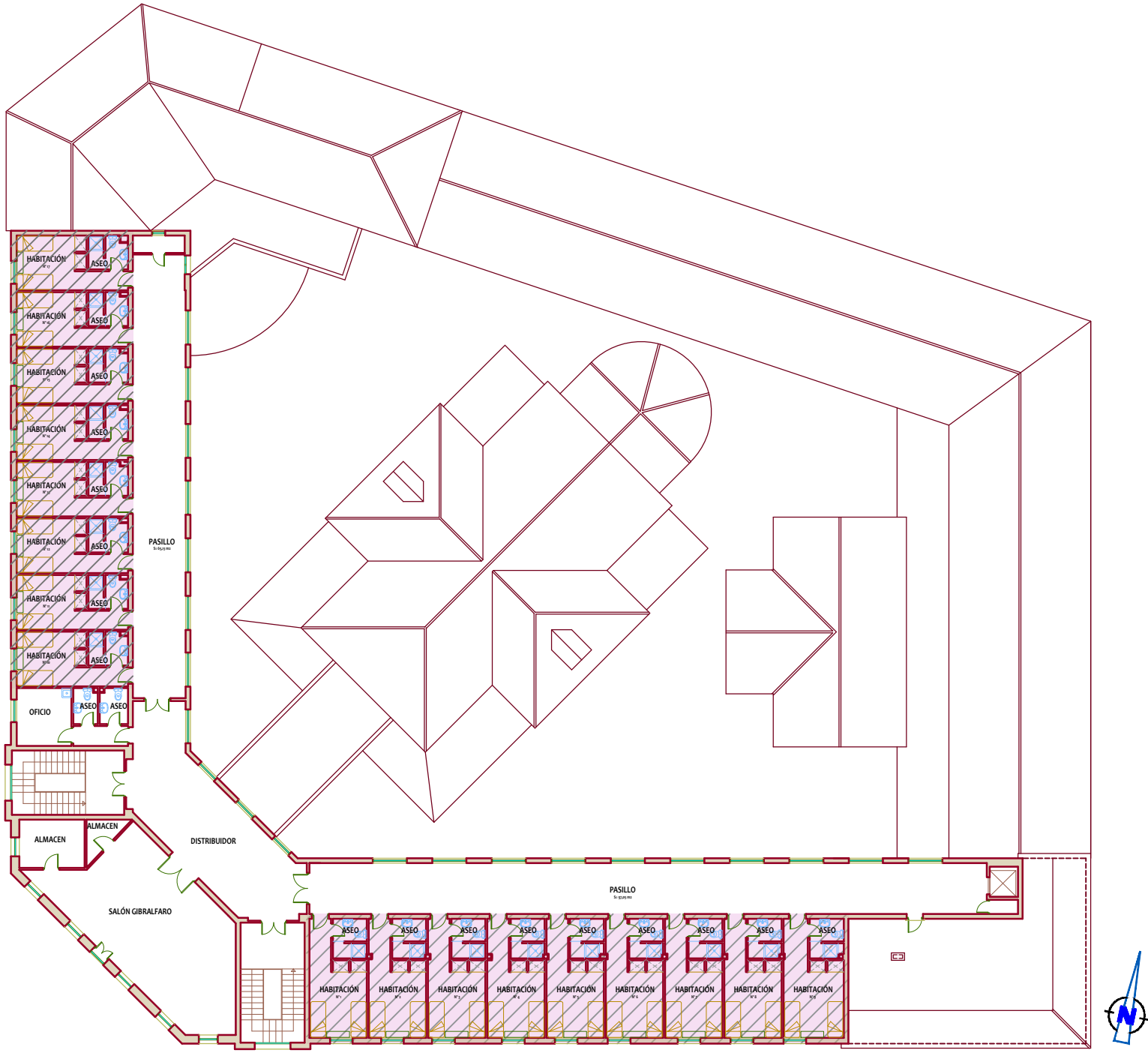
PLANTA SEGUNDA
