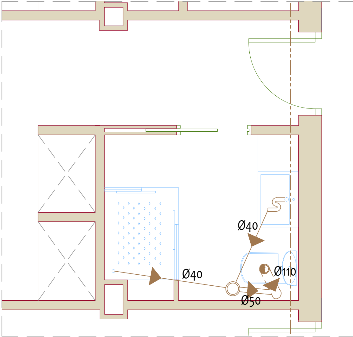
LEYENDA DE SANEAMIENTO
