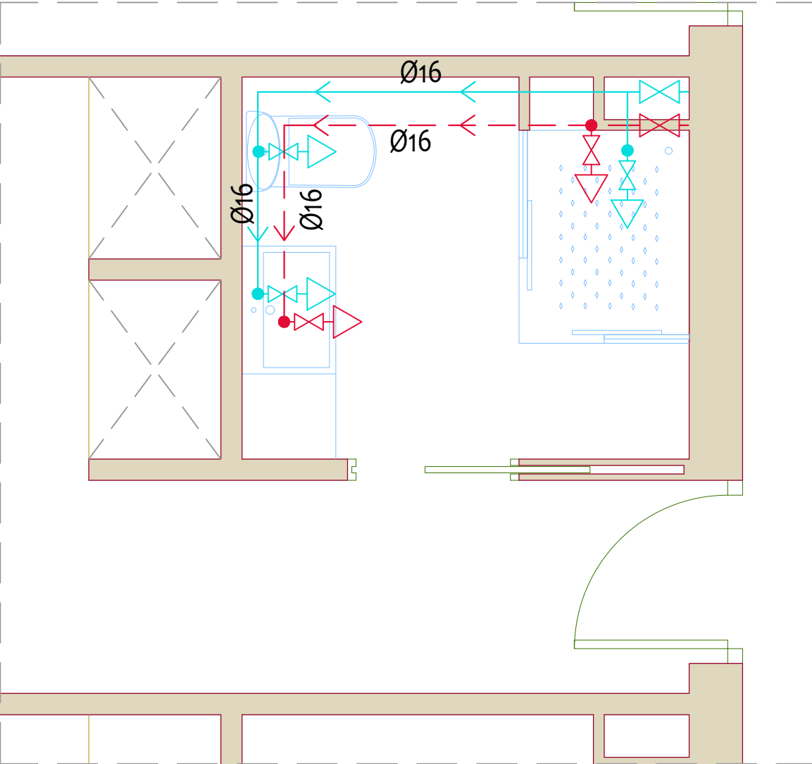
LEYENDA DE FONTANERÍA
