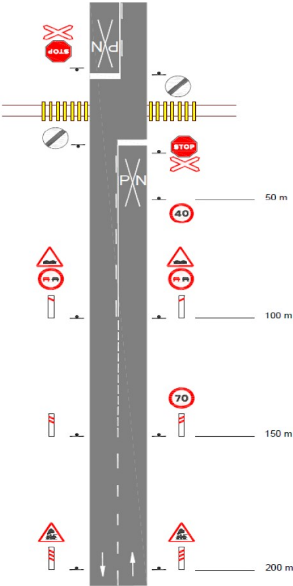
Figura C2. Señalización de paso a nivel sin barreras según la norma 8.1-IC
