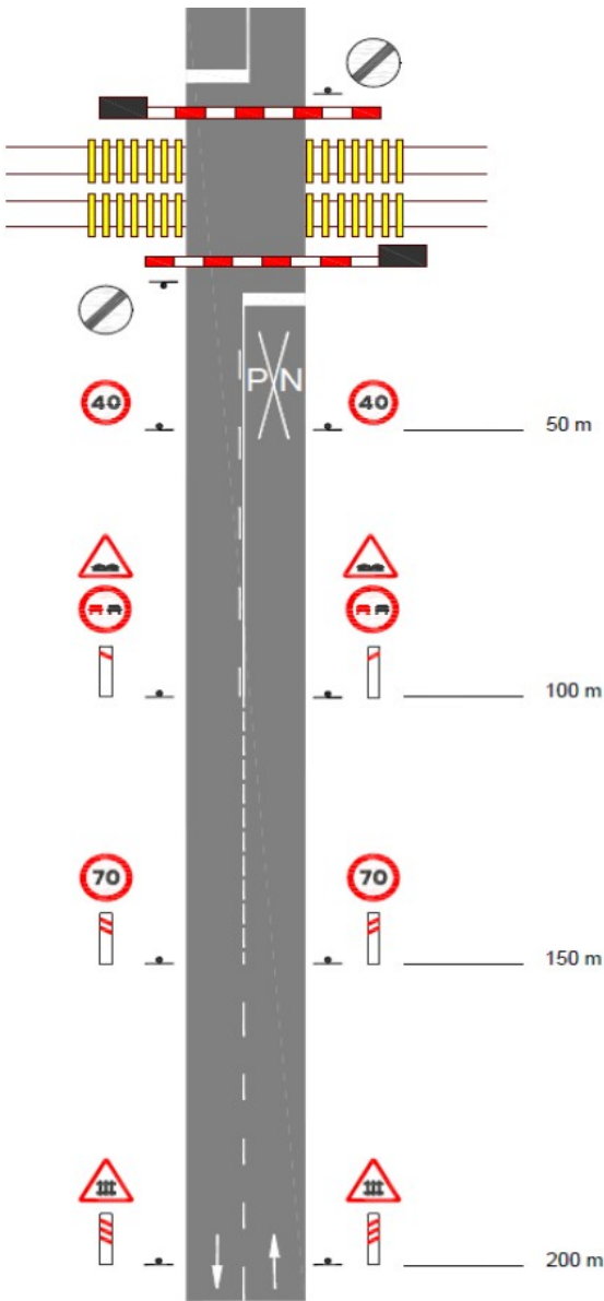
Figura C1. Señalización de paso a nivel con barreras según la norma 8.1-IC
