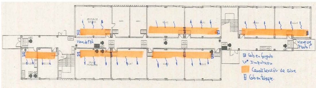
Planta baja
