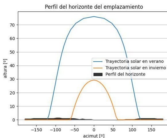
Ilustración 63. Perfil del horizonte lejano del emplazamiento y trayectoria solar en los solsticios.
