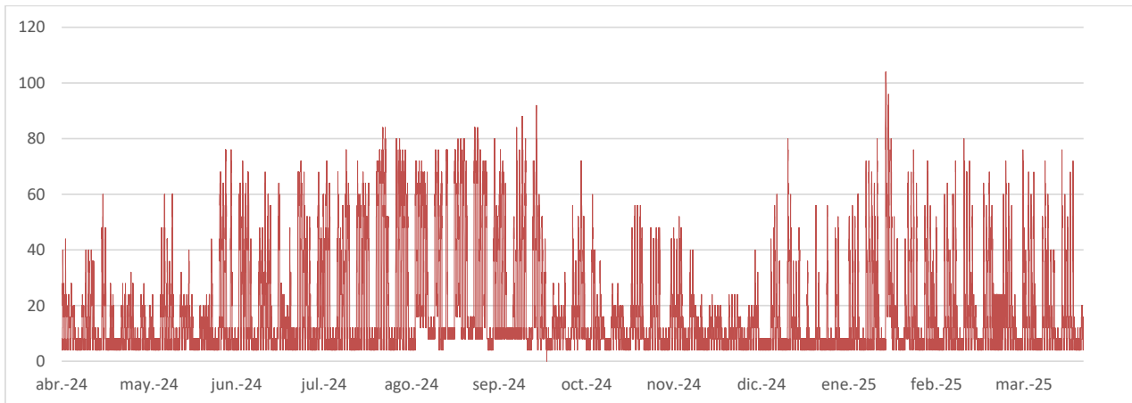
Ilustración 46 Potencia activa demandada por el centro durante el último año
