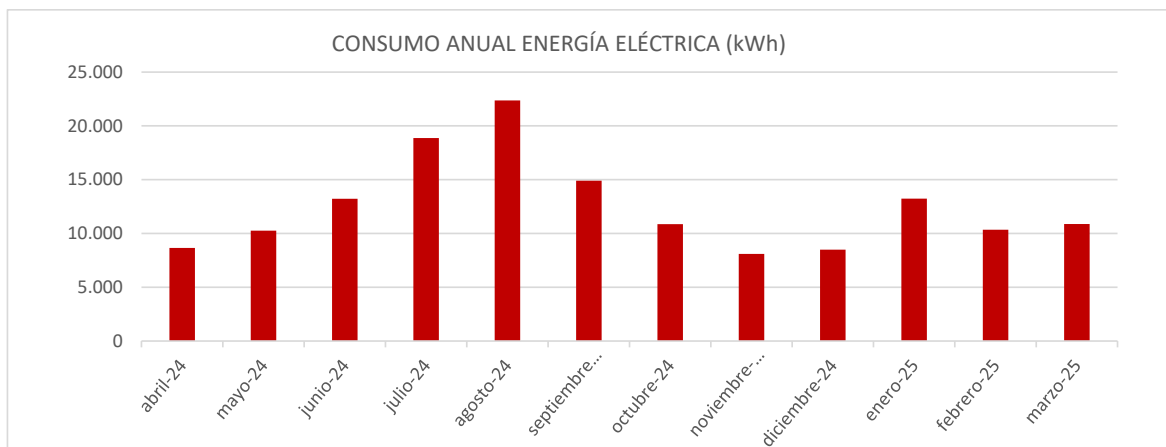
Ilustración 50 Consumo de energía eléctrica del edificio 23-24 (kWh)
