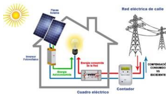
Ilustración 65. Esquema de instalación fotovoltaica conectada a red para autoconsumo.
