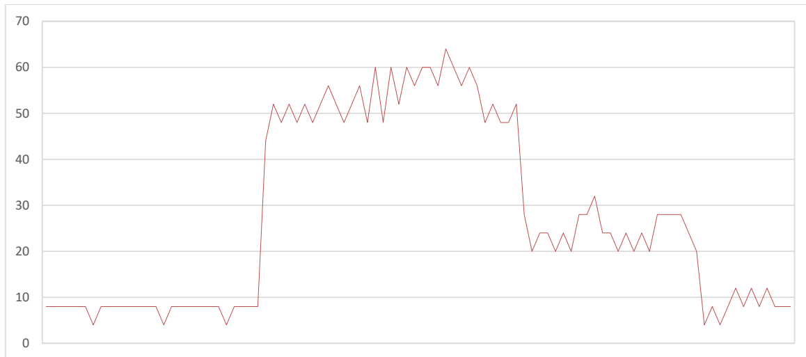
Ilustración 48 Consumo de potencia activa demandado por el centro de salud durante un día laboral
