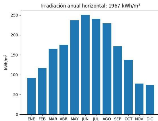
Figura 1 Distribución mensual de la irradiación global sobre el plano horizontal.
