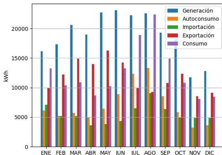
Figura 2 Balance mensual de energía del sistema.
