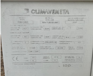
Ilustración 12 Placa de características
