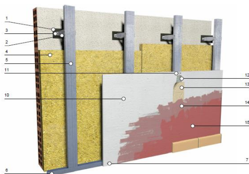
Ilustración 57 Trasdosado autoportante
