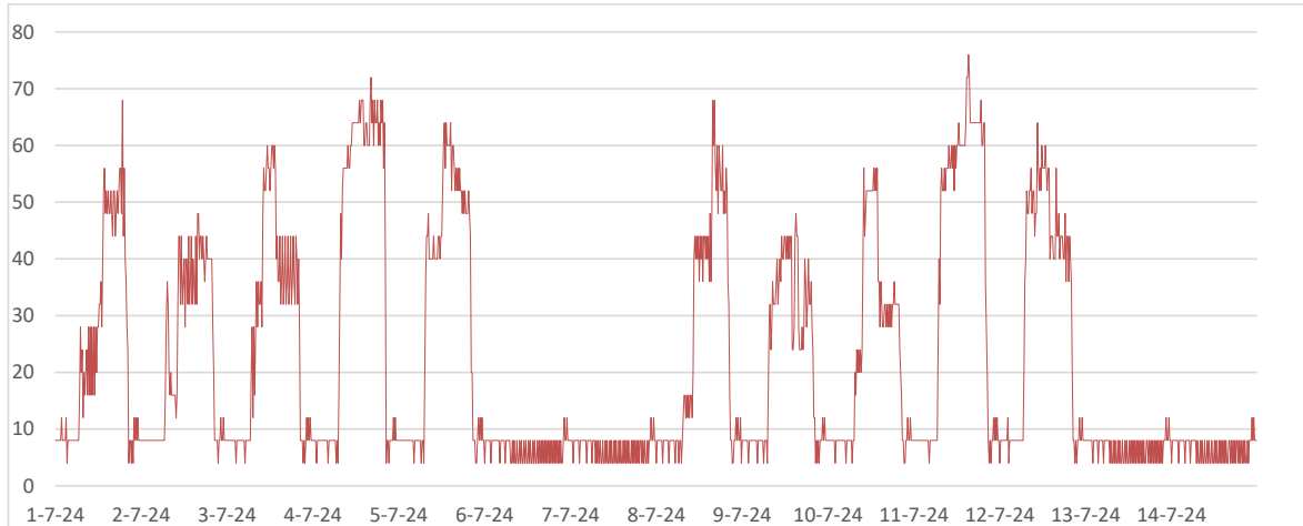
Ilustración 47 Potencia activa demandada por el centro durante un periodo de dos semanas durante el mes de julio
