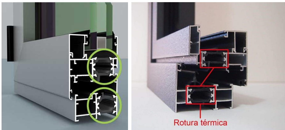
Ilustración 54 Carpintería de aluminio con vidrio doble
