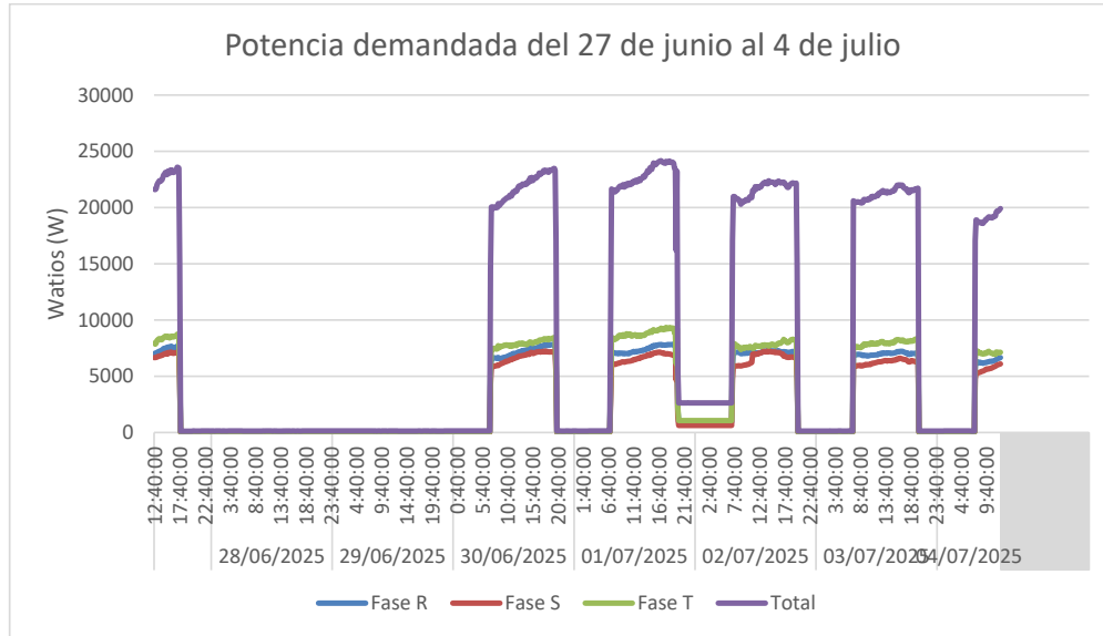
Gráfico 2 Potencia demandada del 27 de junio al 4 de julio en maquinaria de clima
