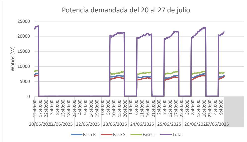
Gráfico 1 Potencia demandada del 20 al 27 de junio en maquinaria de clima
