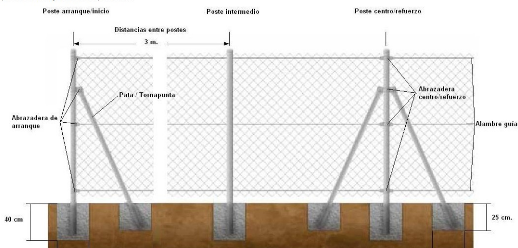
Esquema de montaje vallado Simple Torsión
