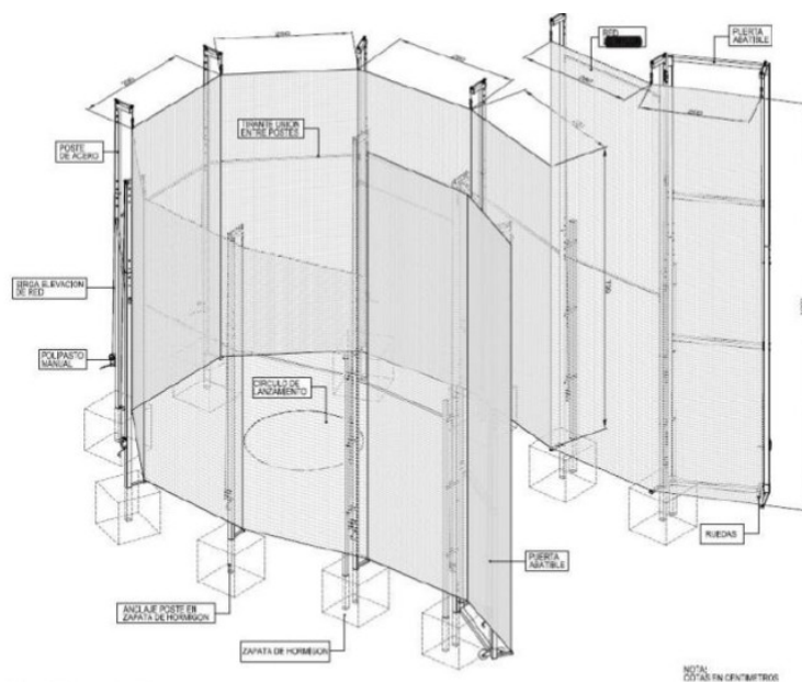
Diseño de Jaula propuesta
