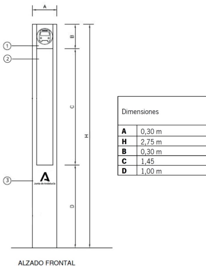
Imagen 15: Alzado poste indicativo de parada
