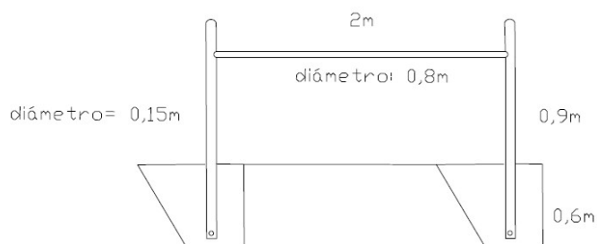
DETALLE DEL VALLADO DE MADERA ENCASTRADO
