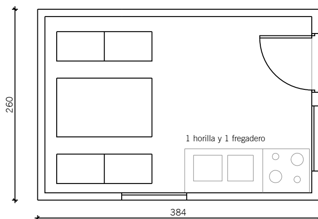
CASETA PREFABRICADA COMEDOR. ALTURA LIBRE 2.50 M
