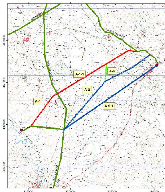
Plano con las alternativas de trazado de la línea eléctrica proyectada.
