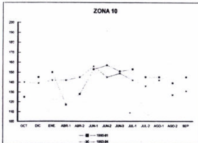
FIGURA 10: VALORES DEL INDICE DE VEGETACION IMAGEN NOAA11-AVHRR
