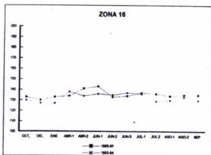
FIGURA 16: VALORES DEL INDICE DE VEGETACION IMAGEN NOAA11-AVHRR
