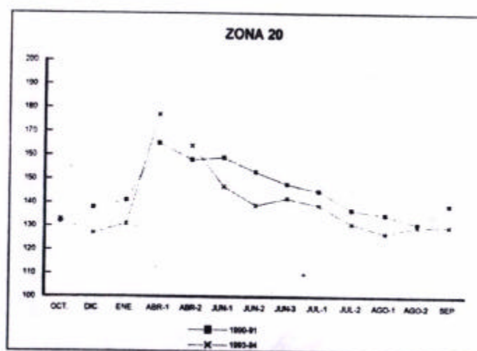
FIGURA 20: VALORES DEL INDICE DE VEGETACION IMAGEN NOAA11-AVHRR
