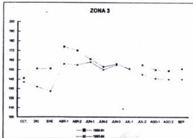
FIGURA 3: VALORES DEL INDICE DE VEGETACION IMAGEN NOAA11-AVHRR
