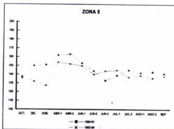
FIGURA 5: VALORES DEL INDICE DE VEGETACION IMAGEN NOAA11-AVHRR
