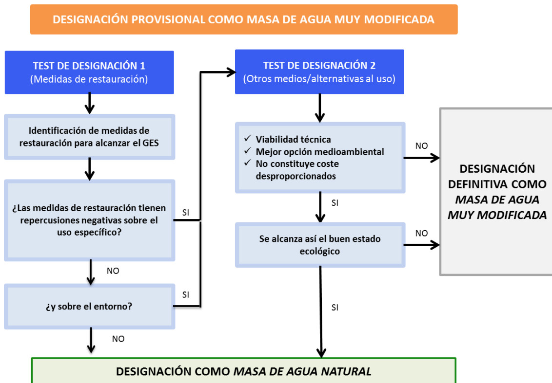
Figura nº 3. Esquema de decisión para la designación definitiva de las masas de agua muy modificadas (MITERD, 2020).
