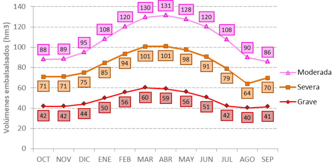
Gráfico 5-20 Umbrales de escasez UTE 03 Sistema de Regulación del Barbate
