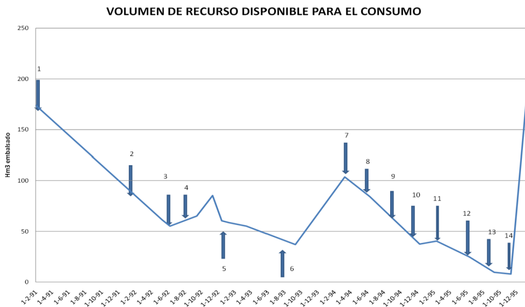
Gráfico 4-4. Evolución del recurso embalsado en la Demarcación durante la sequía 1990 - 1995
