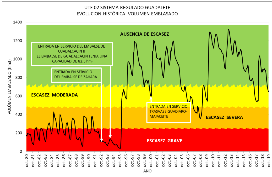
Gráfico 5-18 Evolución histórica del indicador UTE 02 Sistema Regulado del Guadalete
