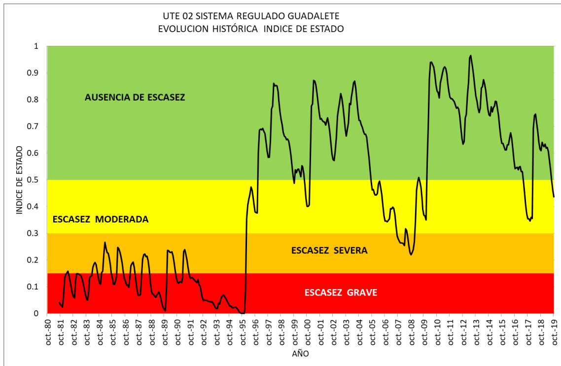
Gráfico 5-19 evolución histórica del Índice de Estado de Escasez UTE 02 Sistema Regulado del Guadalete
