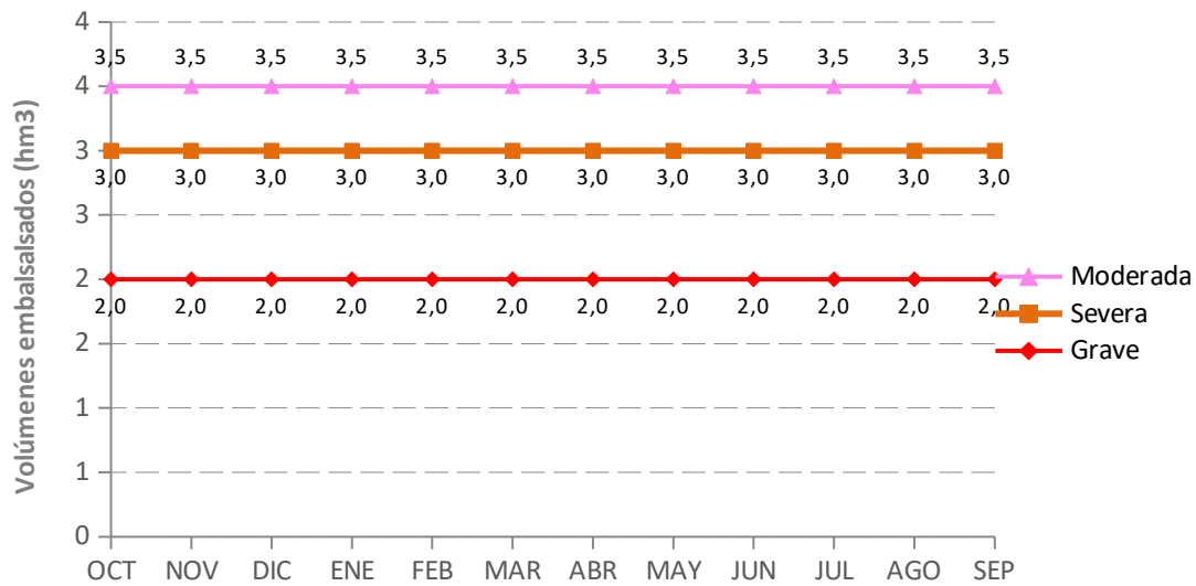
Gráfico 5-23 Umbrales de escasez UTE 04 Abastecimiento a Tarifa
