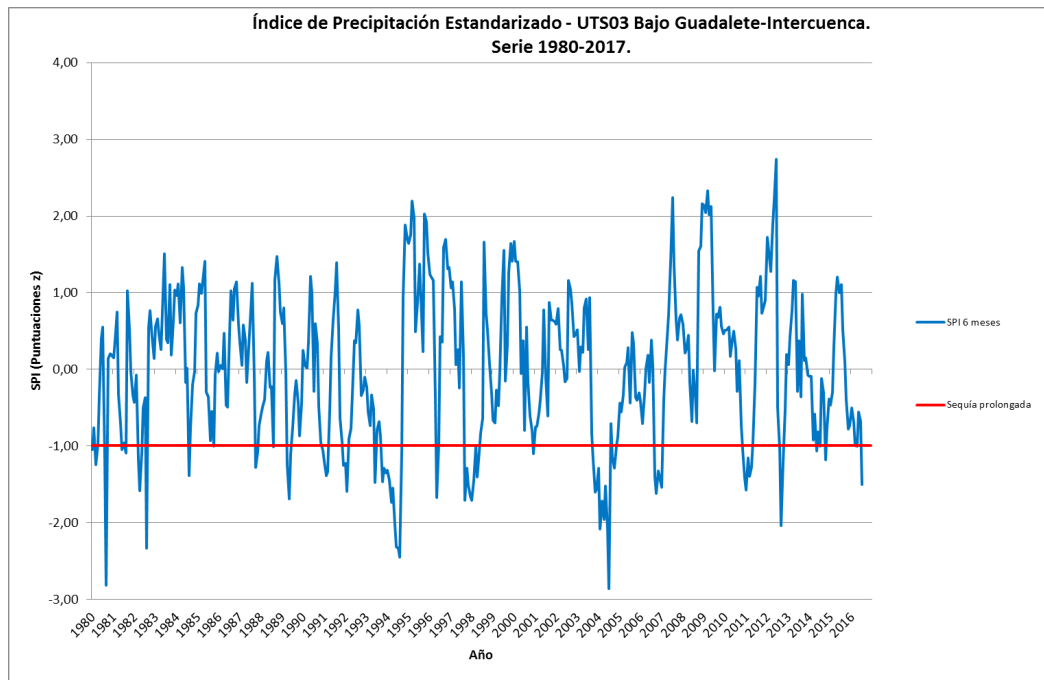
Gráfico 5-5 Evolución del SPI de la UTS03 - Bajo Guadalete-Intercuenca.
