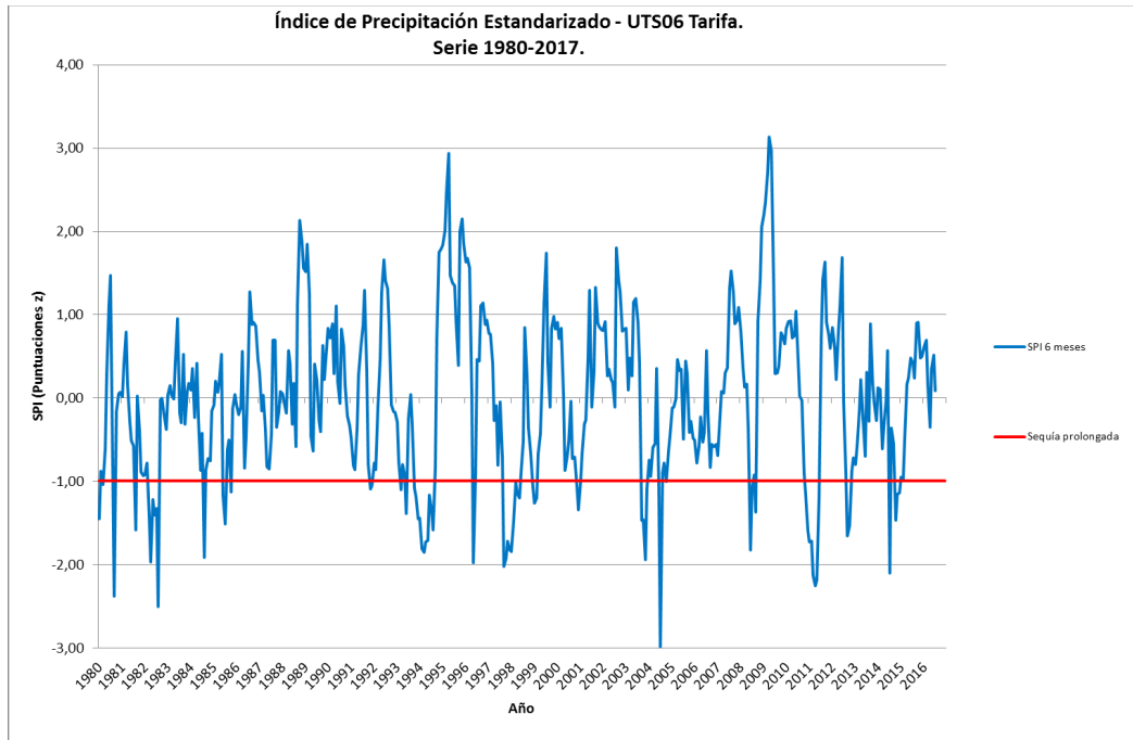
Gráfico 5-11 Evolución del SPI de la UTS06 - Tarifa.
