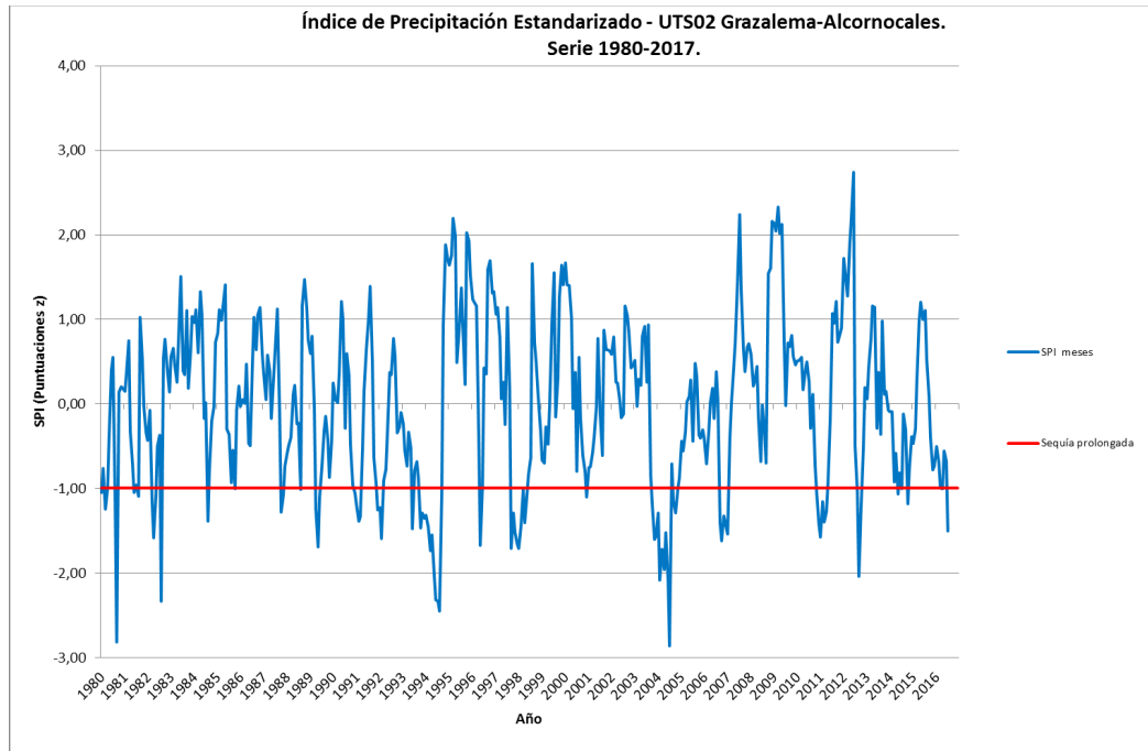
Gráfico 5-3 Evolución del SPI de la UTS02 - Grazelema-Alcornocales.
