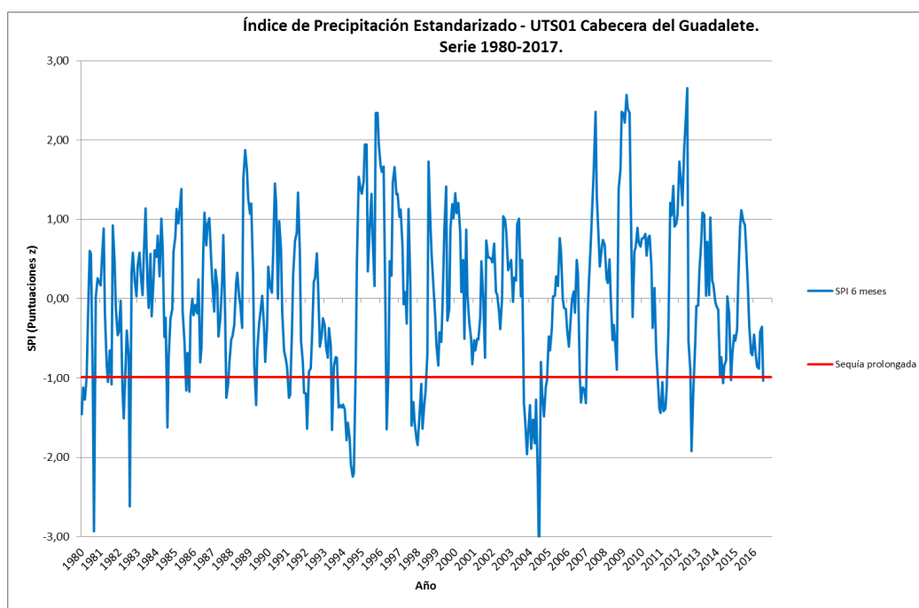
Gráfico 5-1 Evolución del SPI de la UTS01 - Cabecera del Guadalete.
