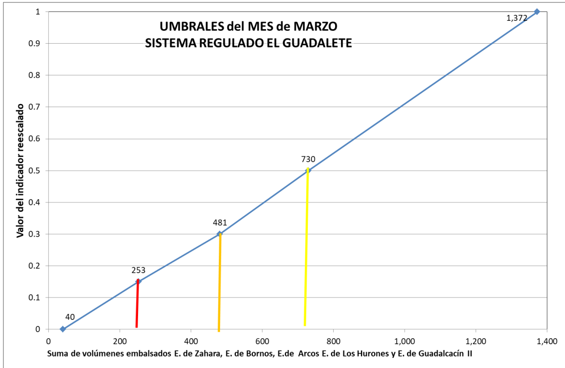
Gráfico 5-13 ejemplo de reescalado del Índice de Estado de Escasez
