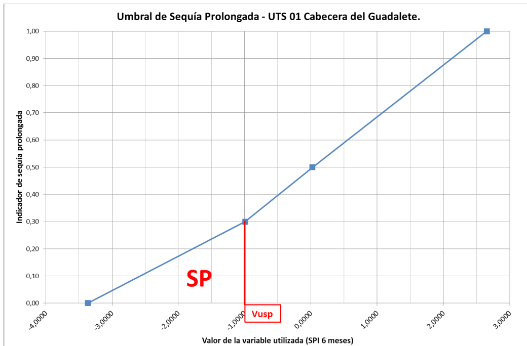
Gráfico 5-2 Umbral de sequía prolongada de la UTS01 - Cabecera del Guadalete.
