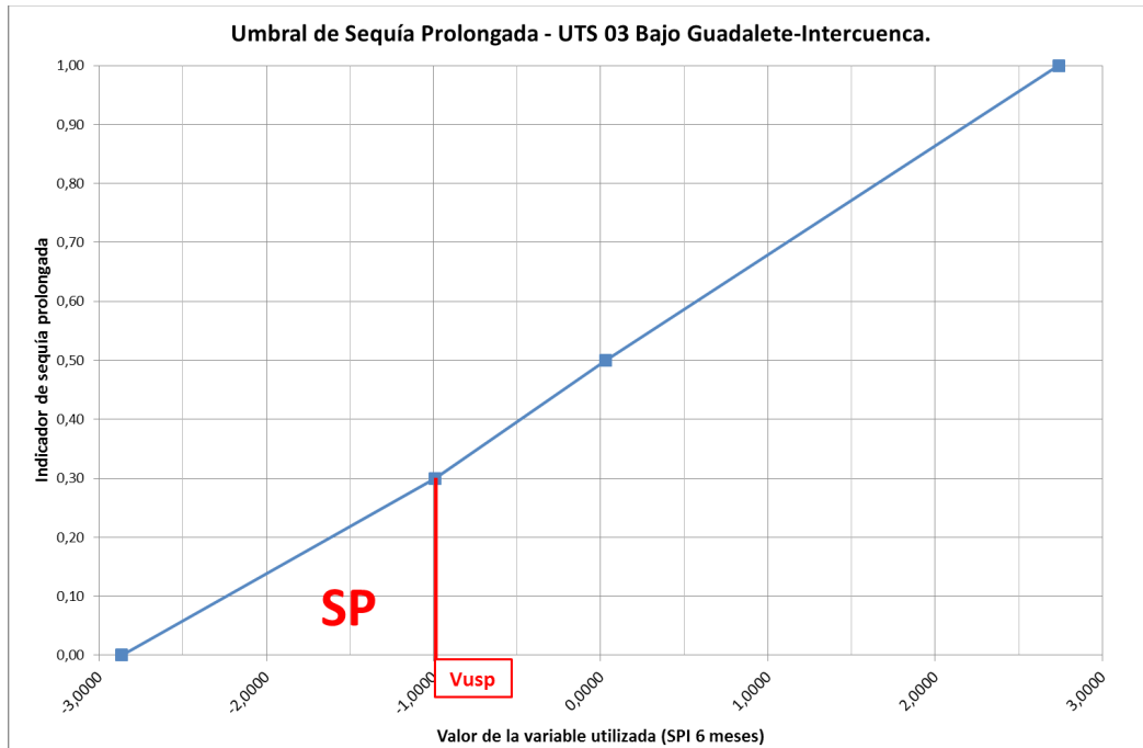
Gráfico 5-6 Umbral de sequía prolongada de la UTS03 - Bajo Guadalete-Intercuenca.
