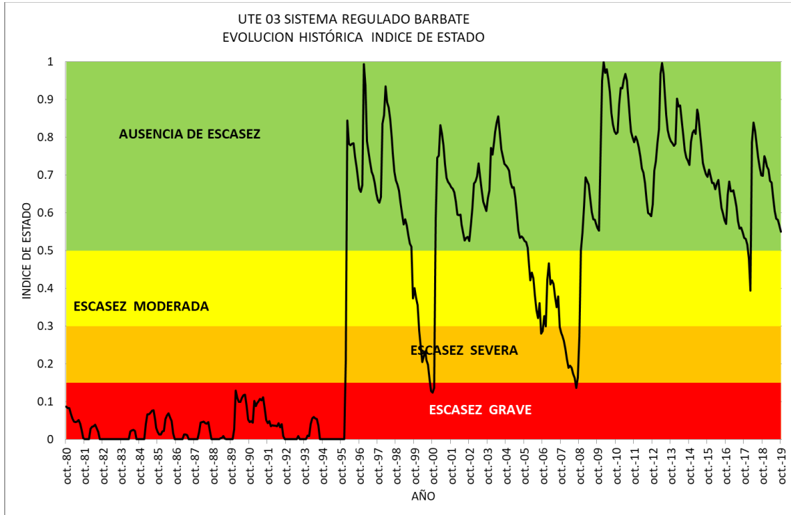
Gráfico 5-22 Evolución histórica del Índice de Estado de Escasez UTE 03 Sistema Regulado del Barbate
