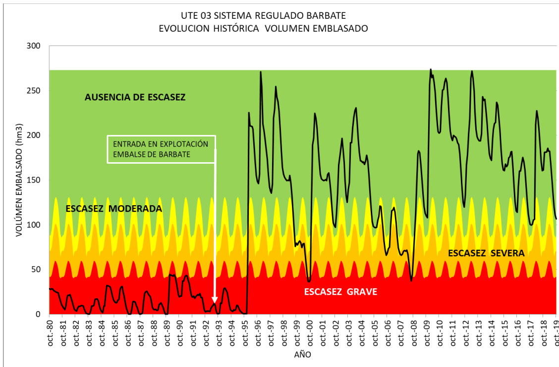
Gráfico 5-21 Evolución histórica del indicador UTE 03 Sistema Regulado del Barbate
