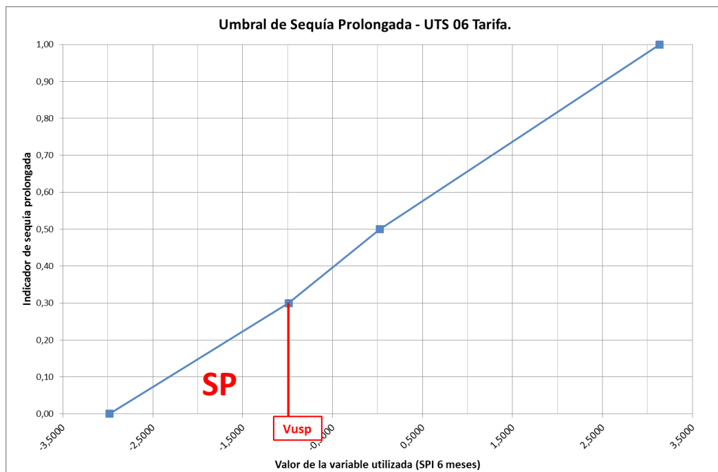
Gráfico 5-12 Umbral de sequía prolongada de la UTS06 - Tarifa.
