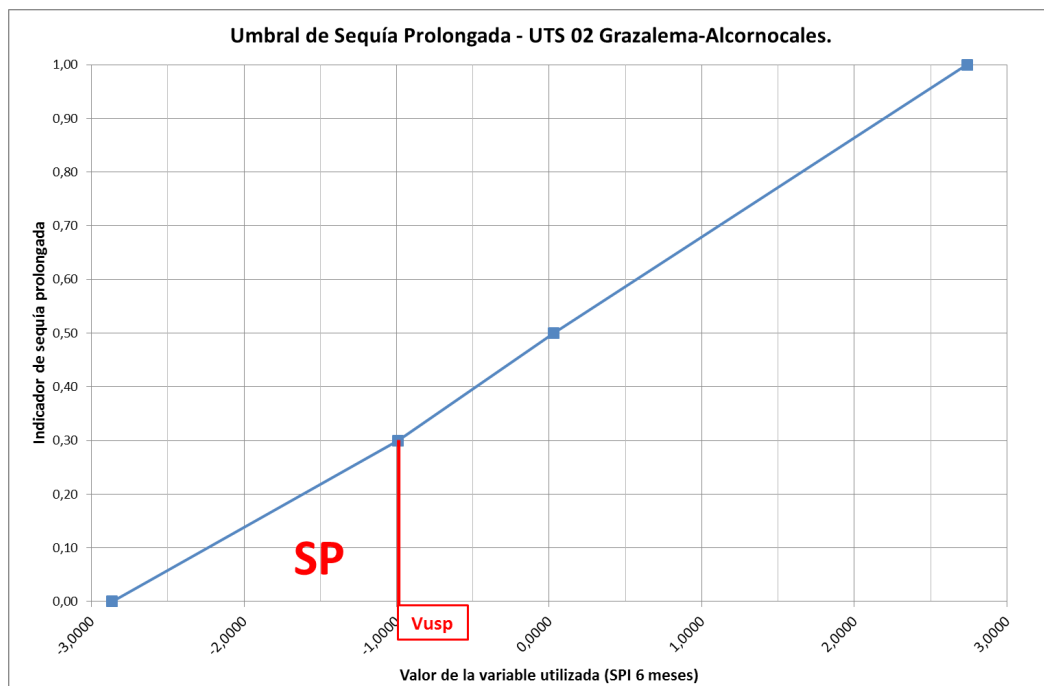
Gráfico 5-4 Umbral de sequía prolongada de la UTS02 - Grazelema-Alcornocales.
