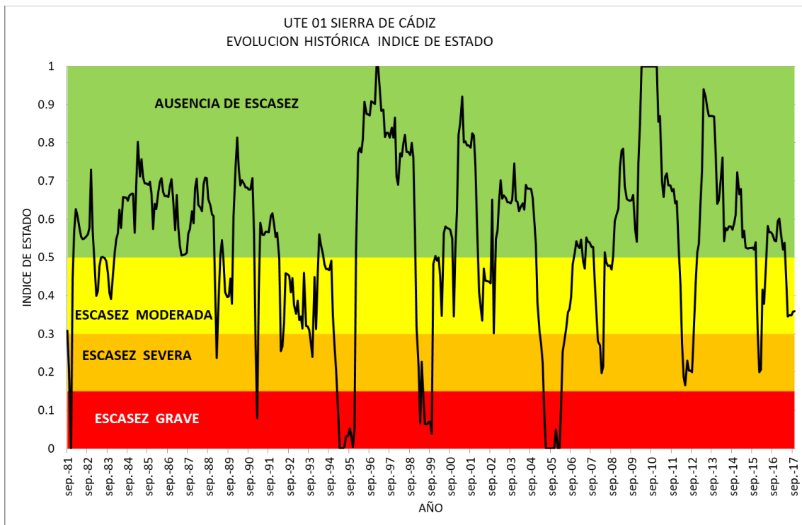
Gráfico 5-16 evolución histórica del Índice de Estado de Escasez UTE 01 Sierra de Cádiz
