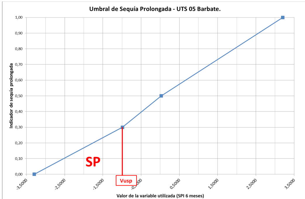
Gráfico 5-10 Umbral de sequía prolongada de la UTS05 - Barbate.
