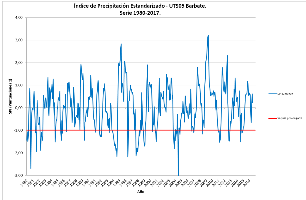
Gráfico 5-9 Evolución del SPI de la UTS05 - Barbate.
