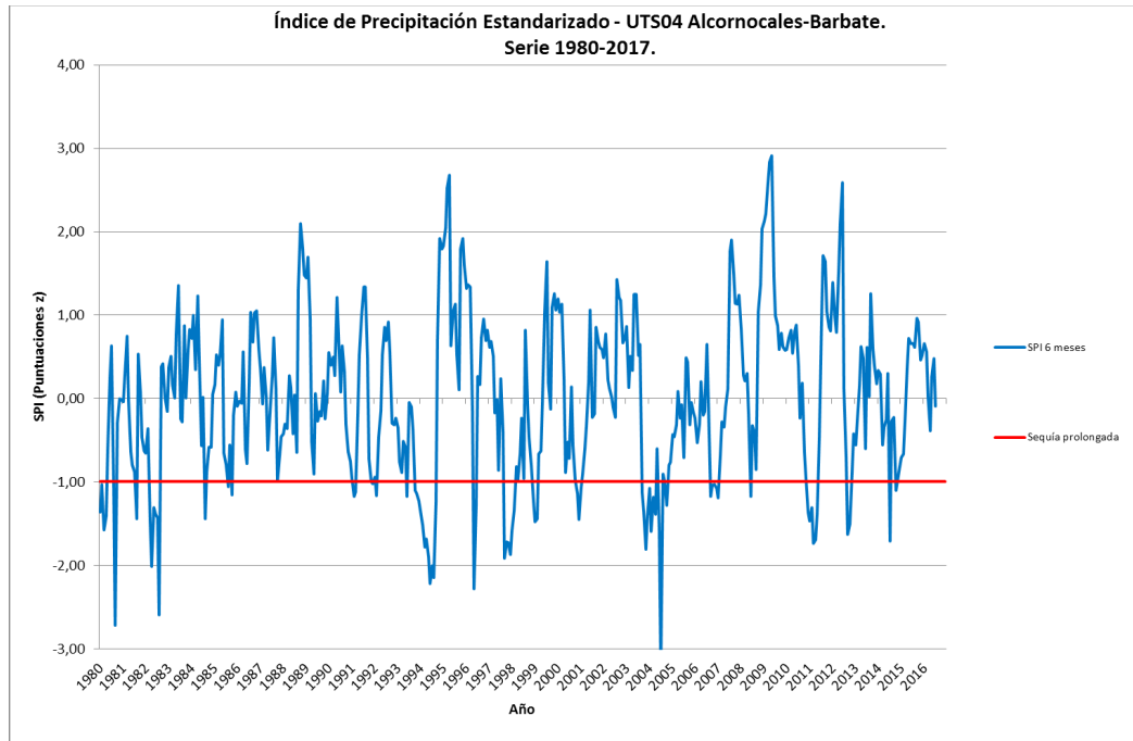
Gráfico 5-7 Evolución del SPI de la UTS04 - Alcornocales-Barbate.
