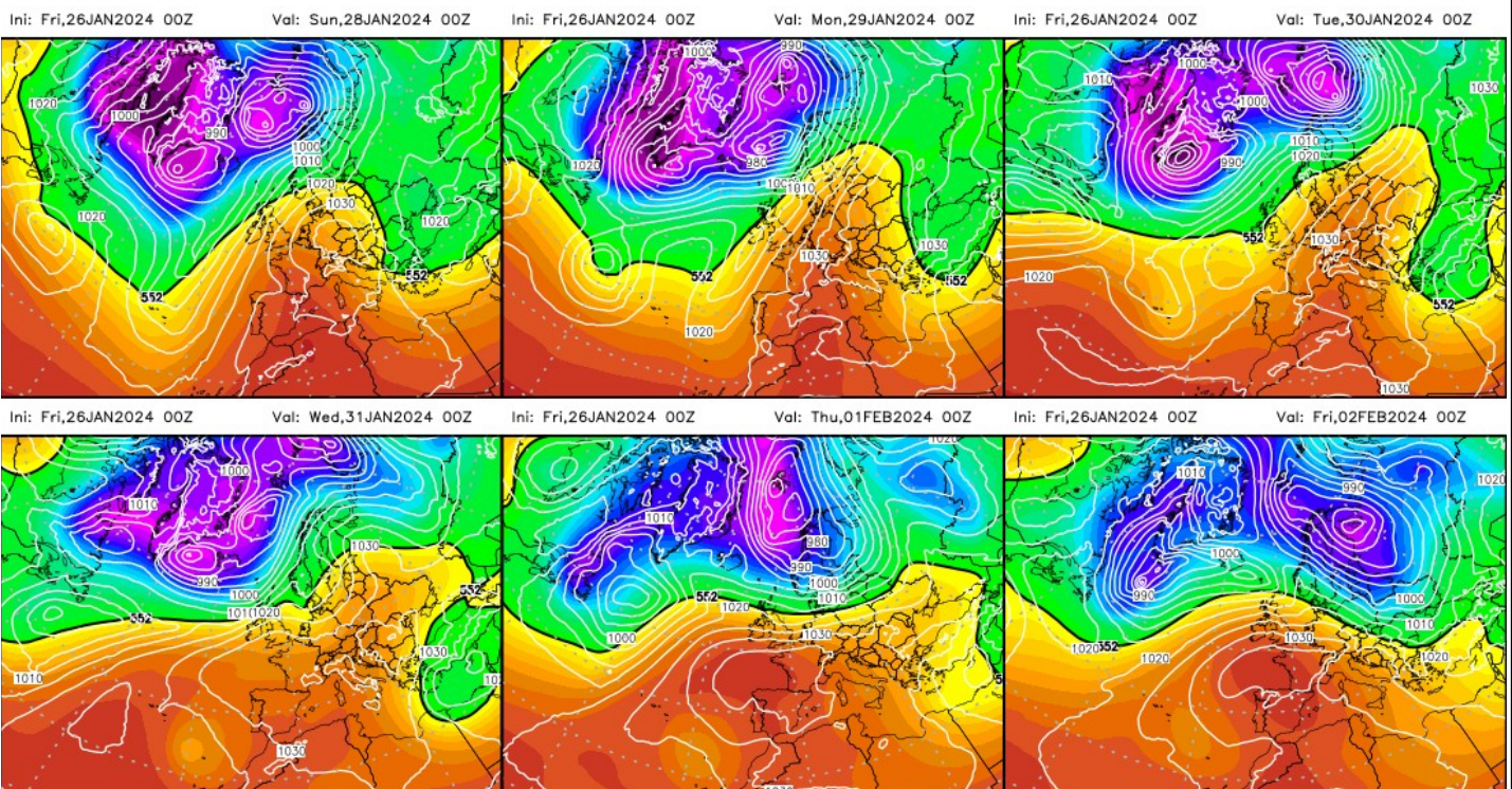
Fig.1: Geopotencial 500 hPa y presión en superficie del 26/01 al 02/02 (modelo: ECMWF, fuente: Wetterzentrale)
