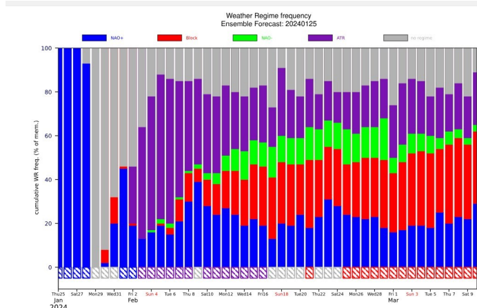
Fig.5: Regímenes meteorológicos euroatlánticos previstos (Fte.: ECMWF)
