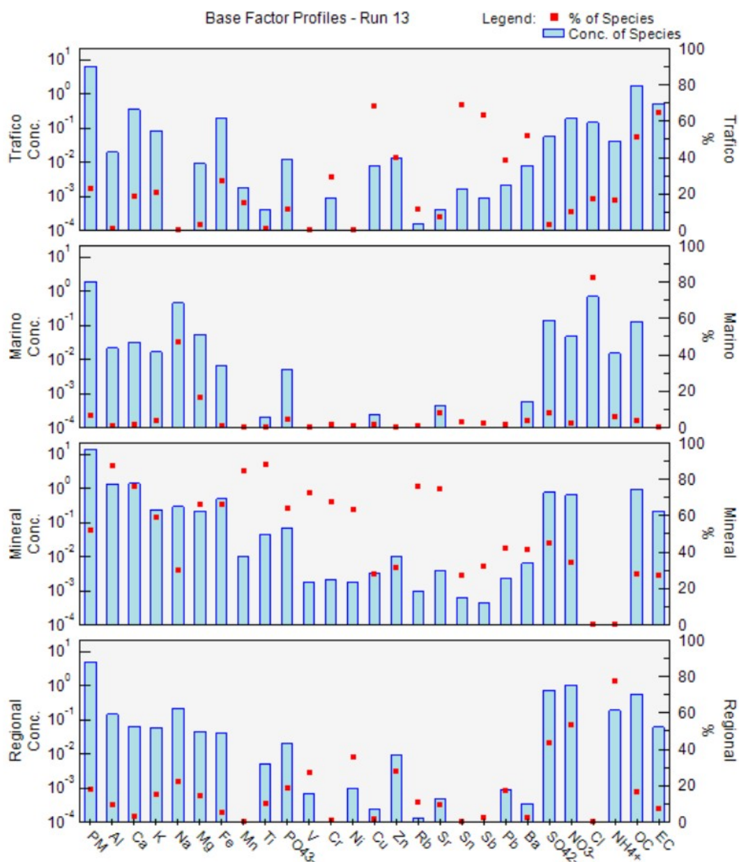
Figura 6.8. Perfil químico de las fuentes de PM 10 (expresado como contribución de elementos mayores y traza en µg/m 3 ) determinadas en la estación de Príncipes en el año 2021
