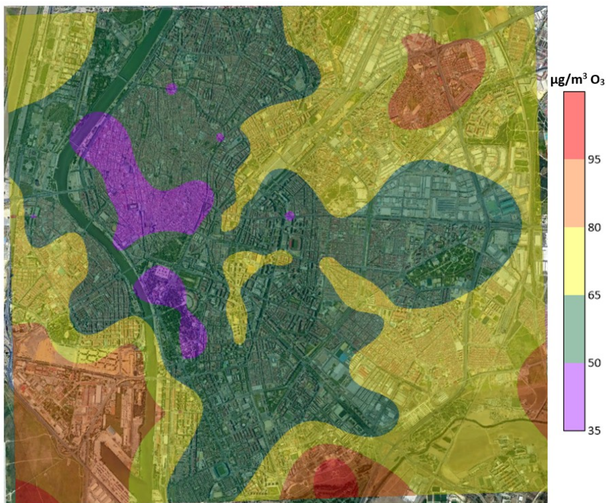
Figura 5.27. Resultados de la campaña de captadores difusivos de O 3 (µg/m³) en Sevilla
