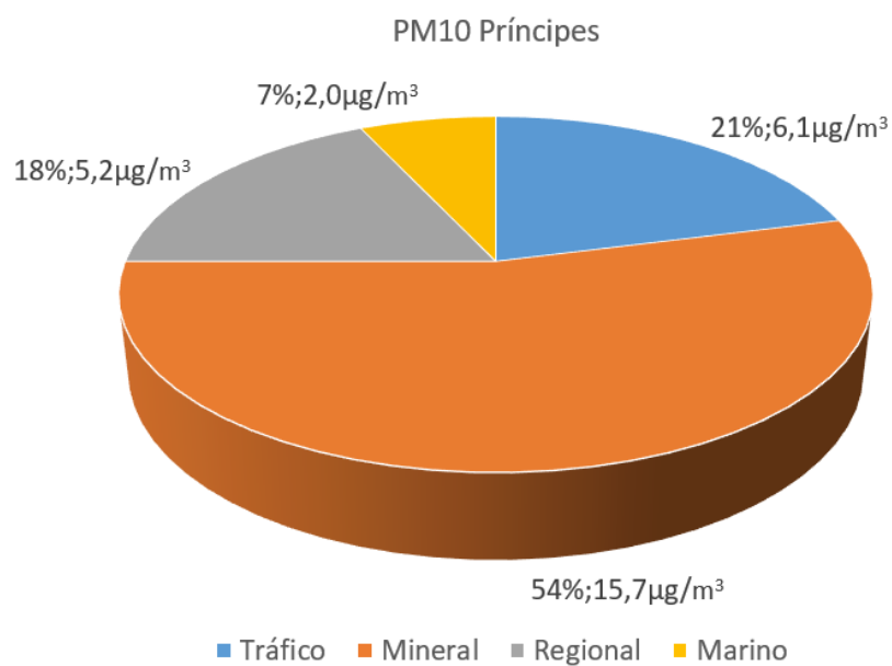
Figura 6.7. Contribución media de fuentes identificadas en el periodo 2021 para \text{PM}_{10} en la estación de Príncipes
