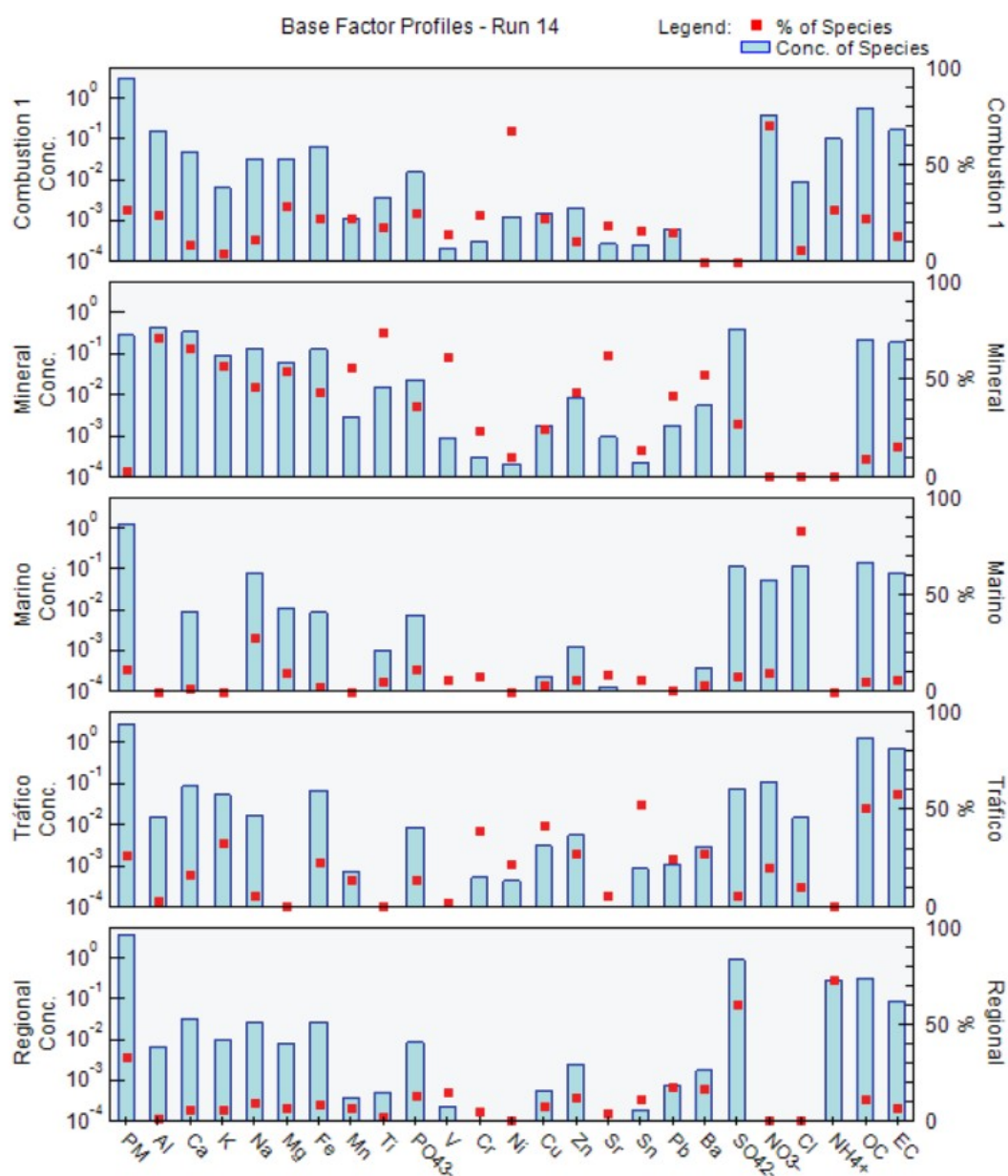
Figura 6.14. Perfil químico de las fuentes de PM_{2.5} (expresado como contribución de elementos mayores y traza en \mu g/m^3 ) determinadas en la estación de Torneo en el año 2021
