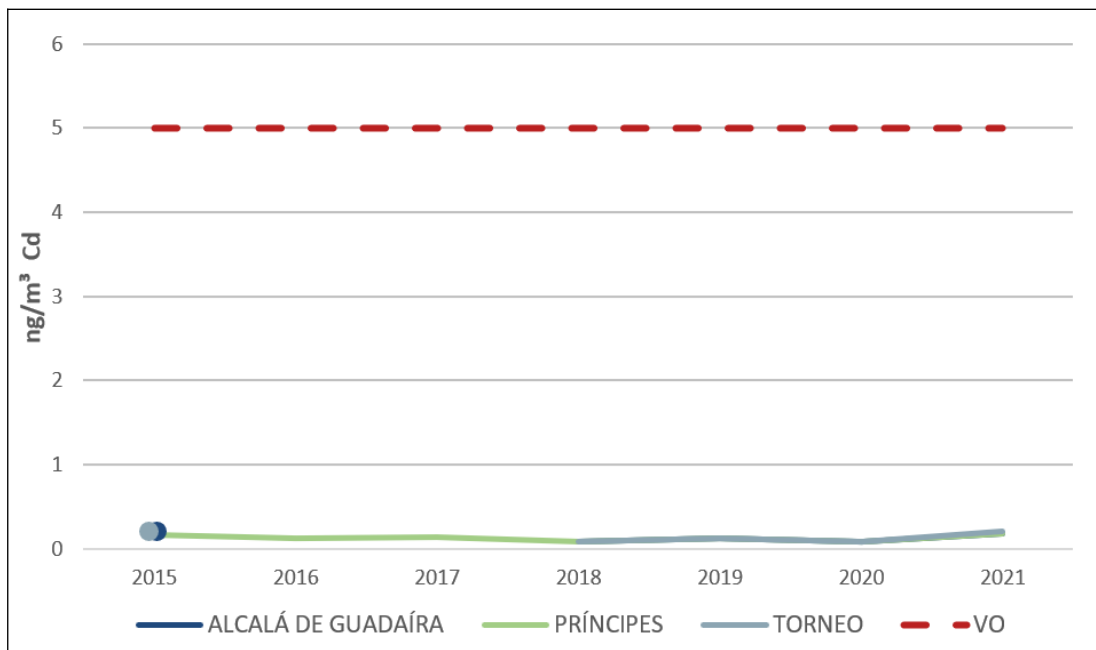
Figura 5.18. Medias anuales de Cd ( \text{ng/m}^3 ) en Sevilla y Área Metropolitana
