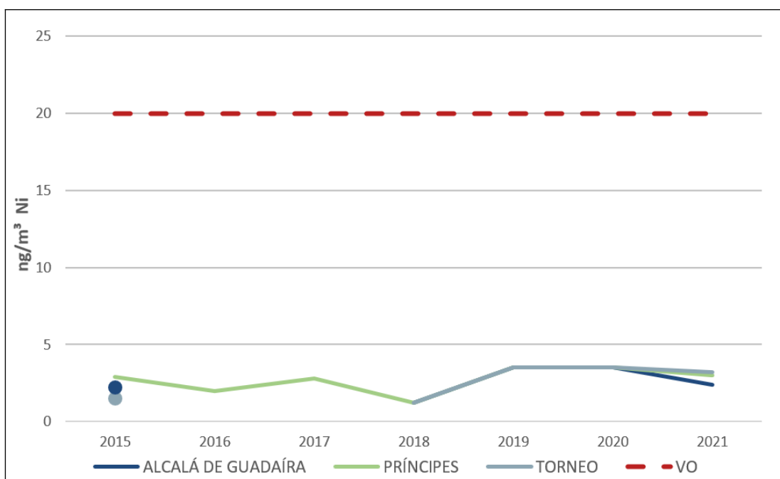
Figura 5.19. Medias anuales de Ni ( \text{ng/m}^3 ) en Sevilla y Área Metropolitana
