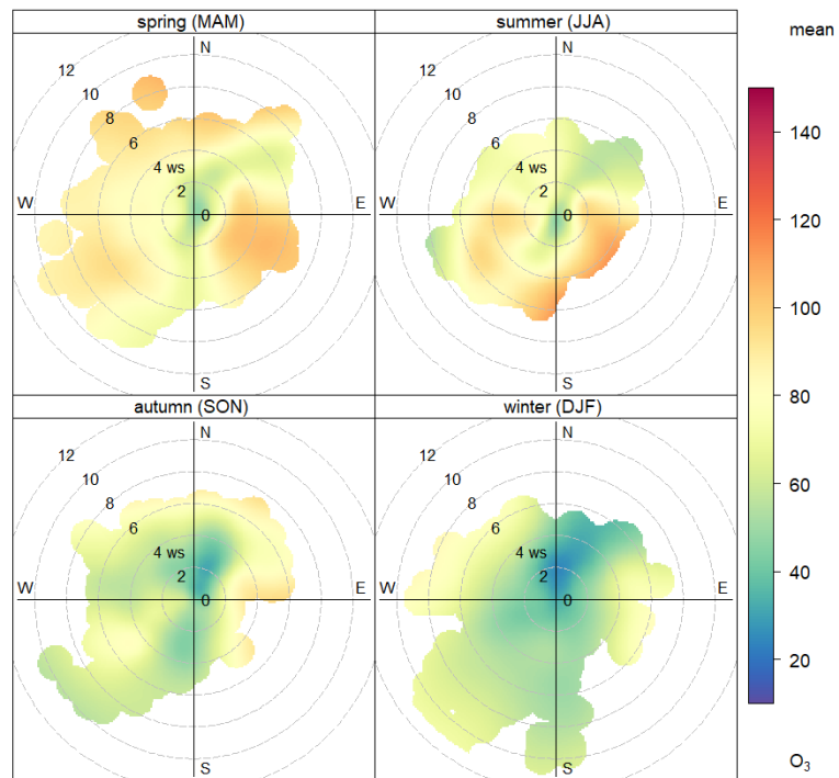
Figura 50. Relación entre los niveles horarios de O_3 y la velocidad y dirección del viento en 2019. Estación Centro
