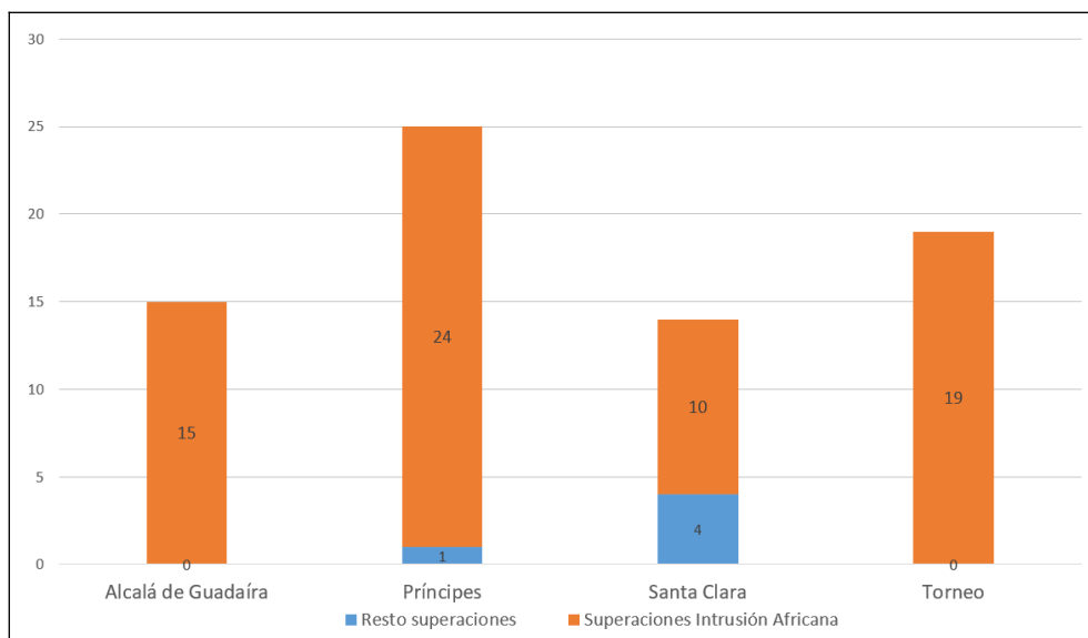
Figura 5.32. Origen y cuantificación del número de superaciones diarias de PM 10 (µg/m³) en 2021 en las estaciones Alcalá de Guadaíra, Príncipes, Santa Clara y Torneo
