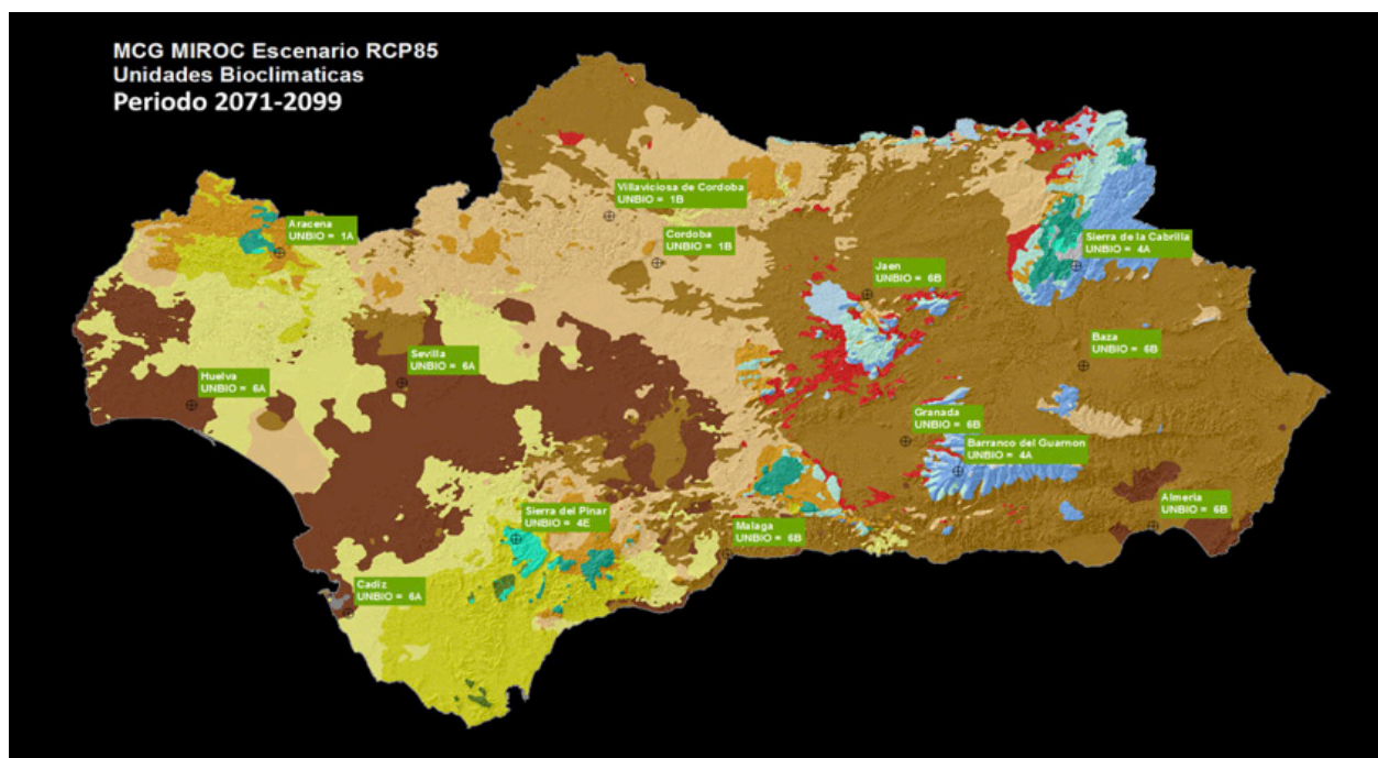
Figura 31. Escenario RCP85 Unidades Bioclimáticas, periodo 1971-2099.
