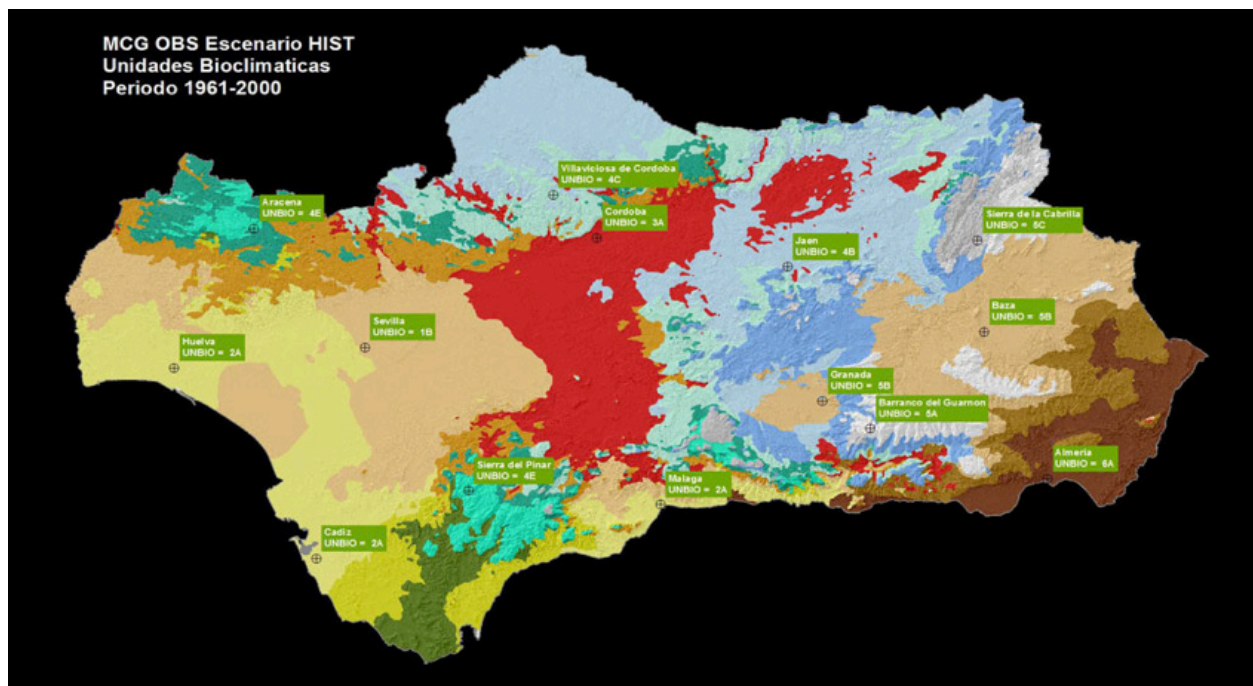
Figura 30. Escenario Histórico Unidades Bioclimáticas, periodo 1961-2000.
