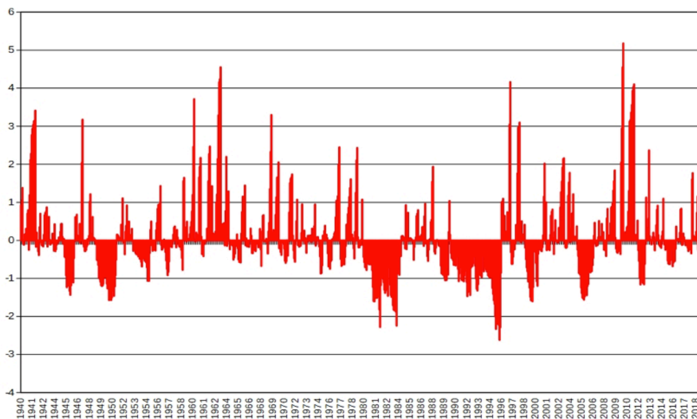
Figura 22. Índice estandarizado mensual de las precipitaciones en Andalucía en la Cuenca del Guadalquivir, 1940-2018.
