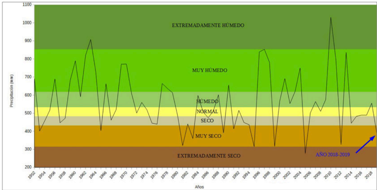
Figura 20. Evolución de las precipitaciones. Fuente: REDIAM 2019.
