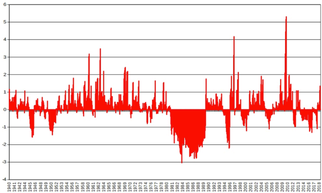
Figura 24. Índice estandarizado mensual de las precipitaciones en Andalucía en la Cuenca Mediterránea Andaluza, 1940-2018.
