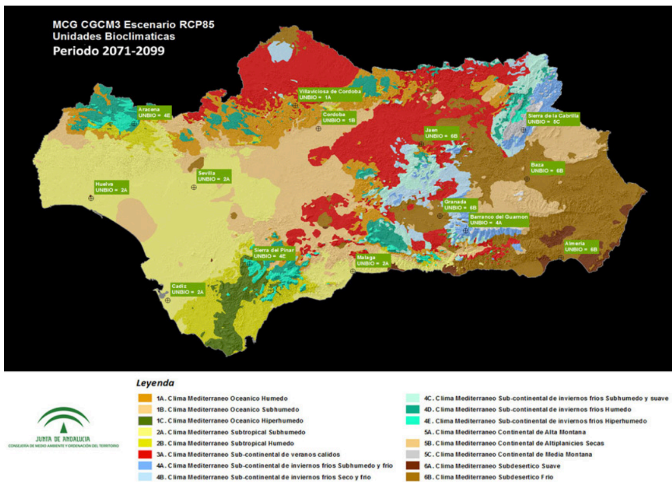
Figura 32. Escenario CGCM3 Unidades Bioclimáticas, periodo 1971-2099.
