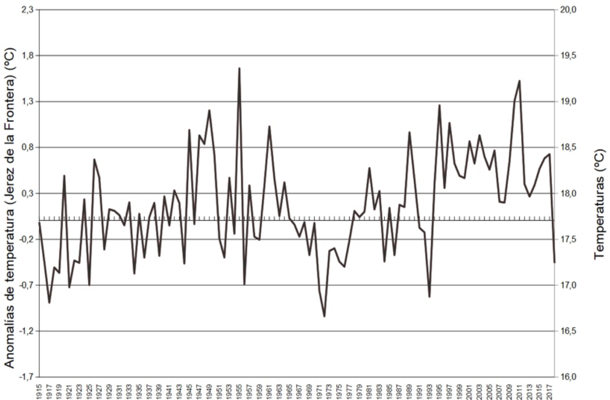
Figura 19. Anomalías de temperatura (Jerez de la Frontera).
