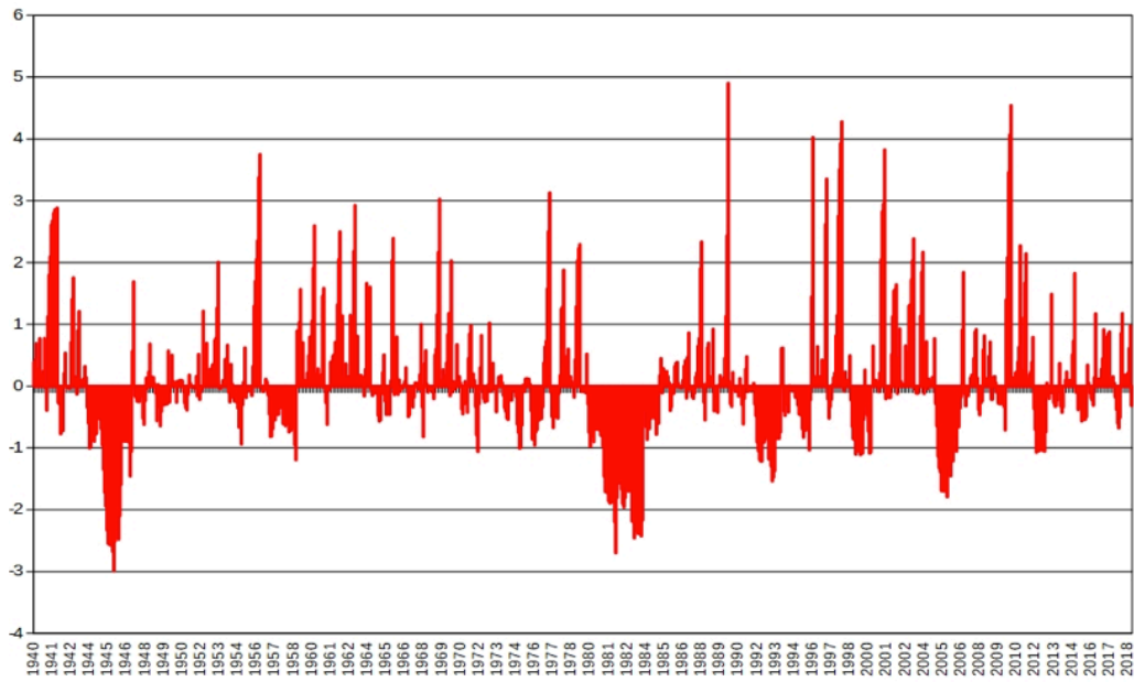
Figura 26. Índice estandarizado mensual de las precipitaciones en Andalucía en la Cuenca del Tinto-Odial-Piedras, 1940-2018.
