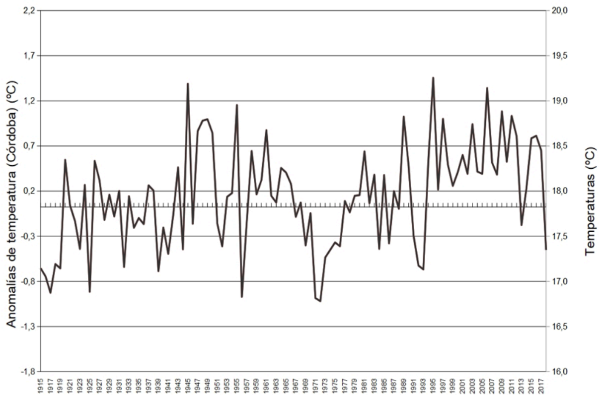
Figura 17. Anomalías de temperatura (Córdoba).
