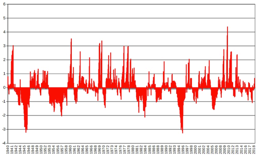
Figura 27. Índice estandarizado mensual de las precipitaciones en Andalucía en la Cuenca del Segura, 1940-2018.
