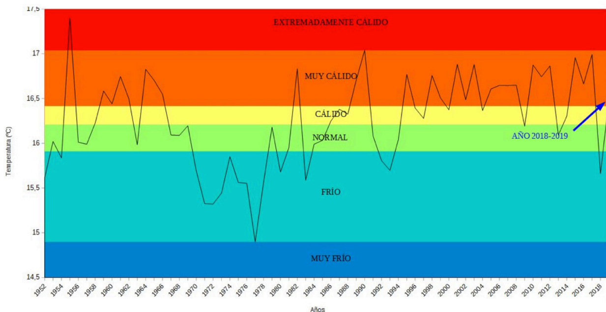
Figura 15. Evolución de las temperaturas, 1952-2018.
